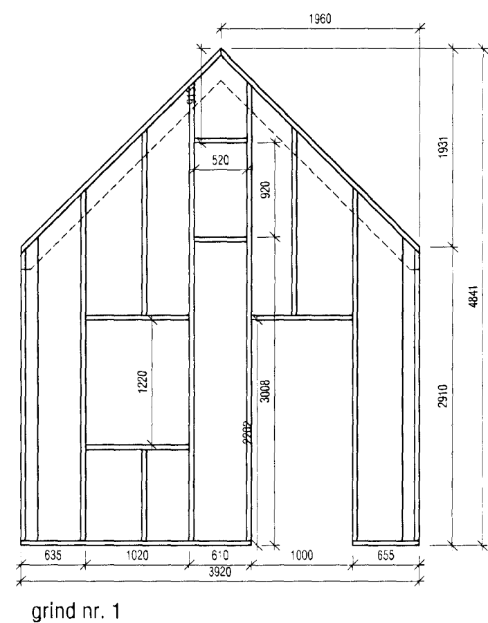
Ásýnd veggjagrinda (utan frá), 1:50
