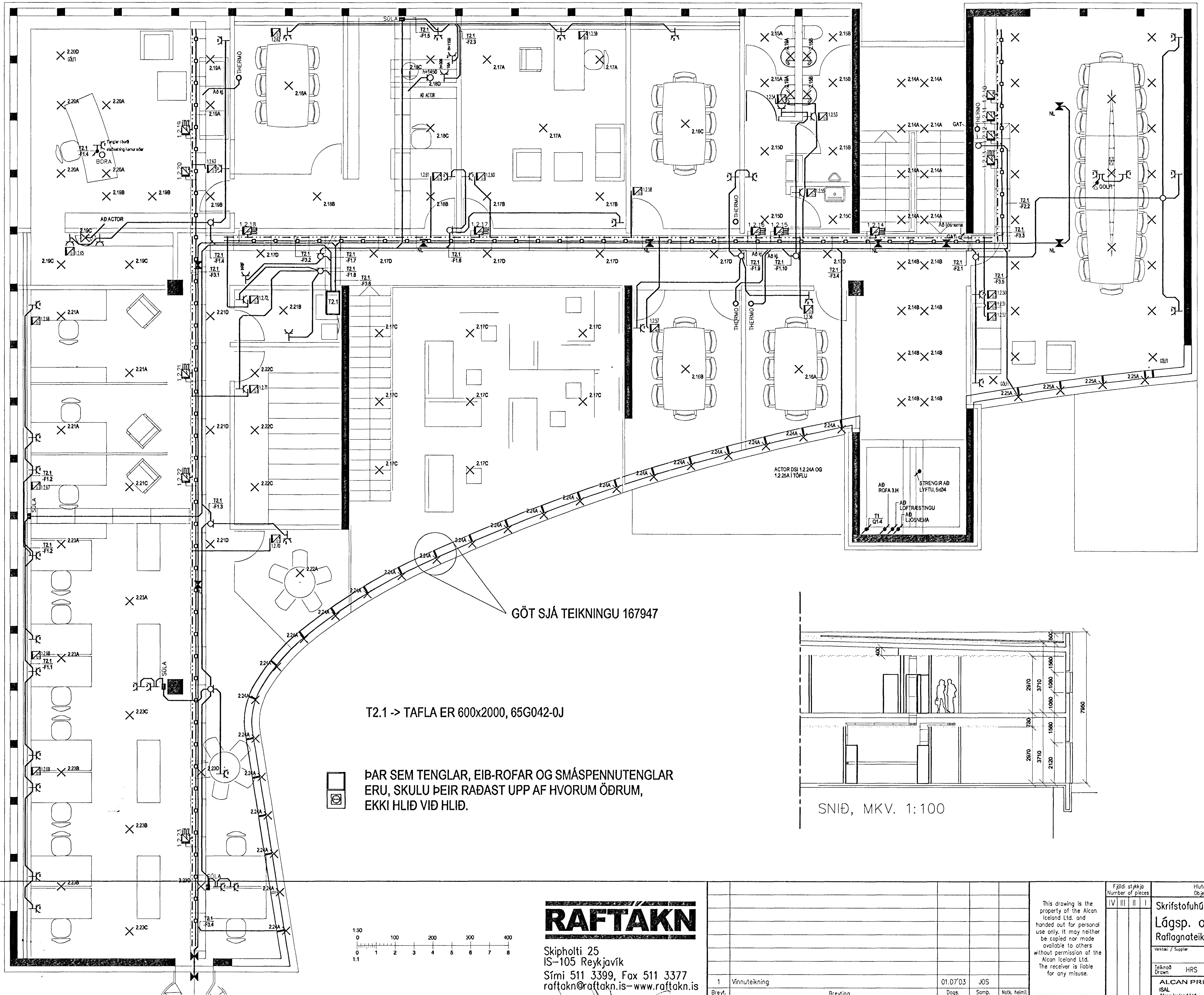
TÆKNIRÝMI 3.HÆÐ
