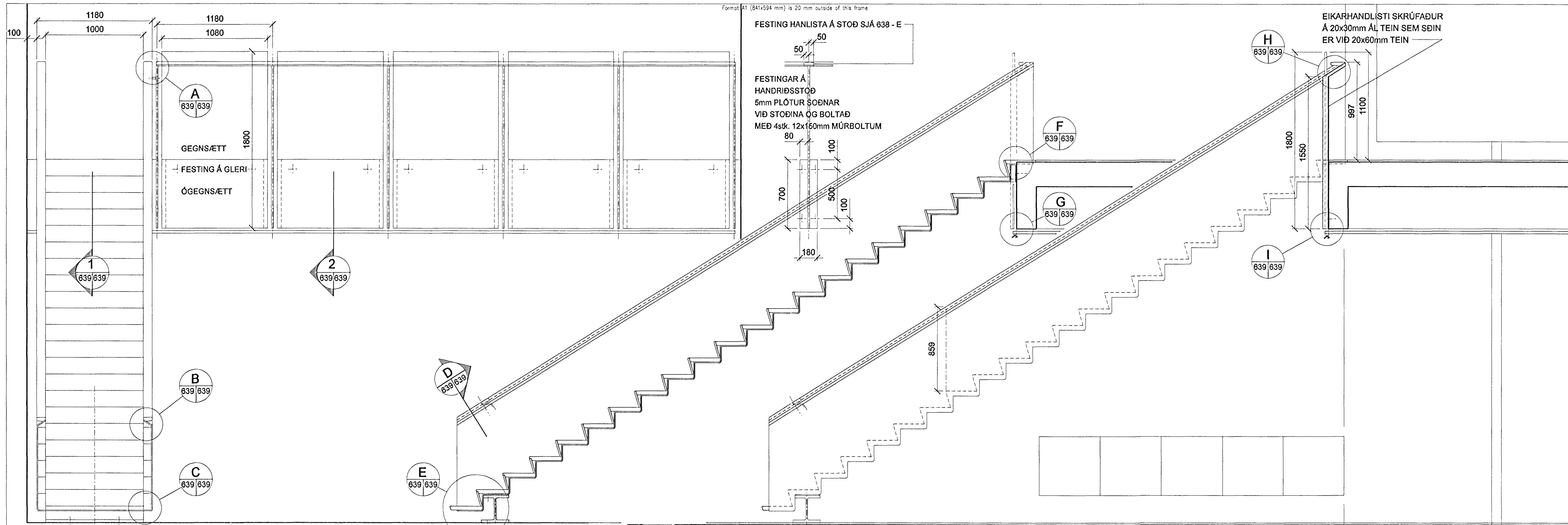
ÚTLIT 1:20 1 SNÍÐ 1:20 2 ÚTLIT 1:20
