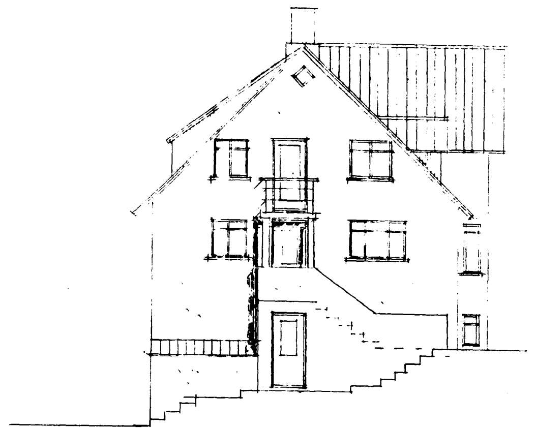
N-V HLIÐ
