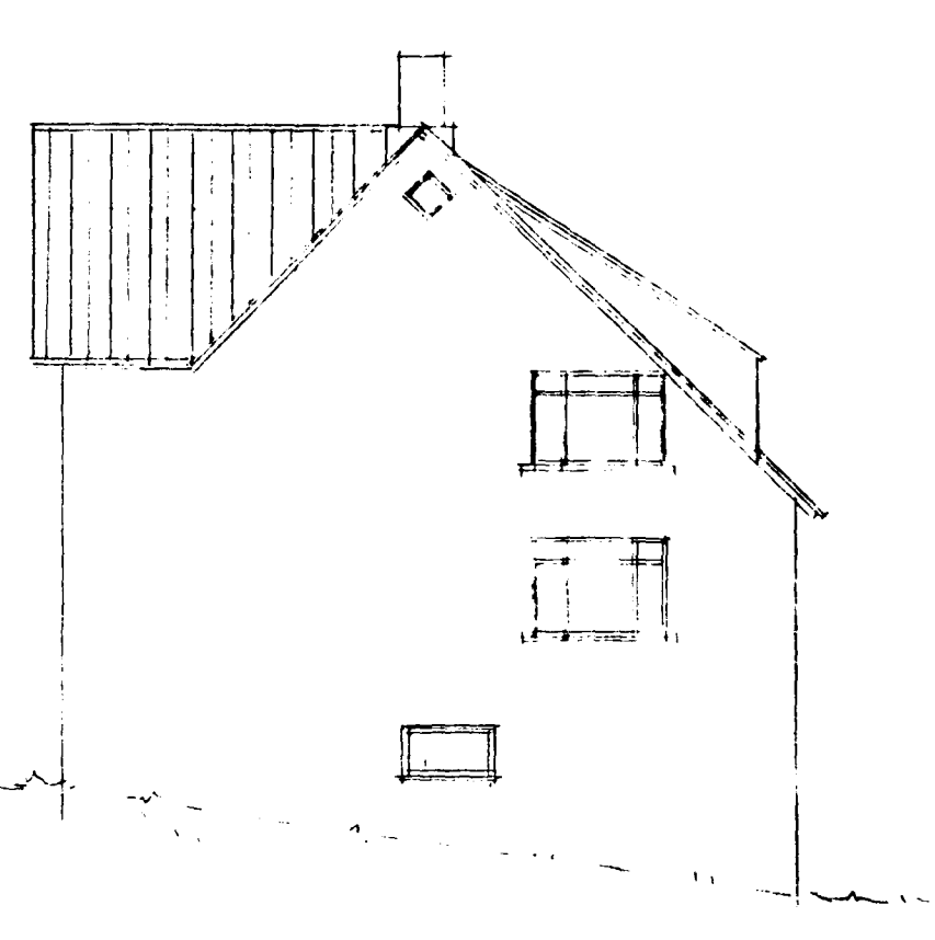
S-A HLIÐ
