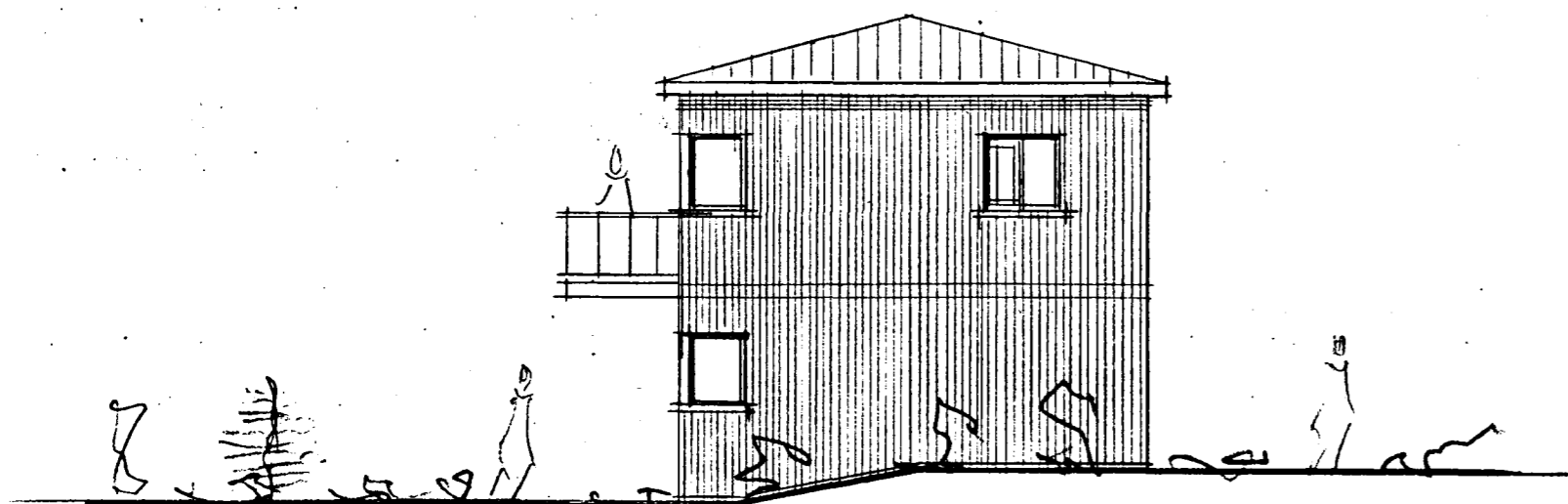
ÚTLIT SUÐUR H=1:100
