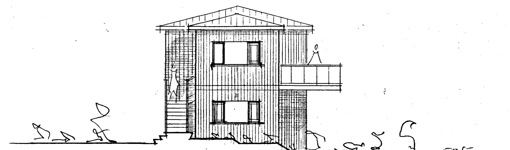
ÚTLIT NORÐUR H=1:100
