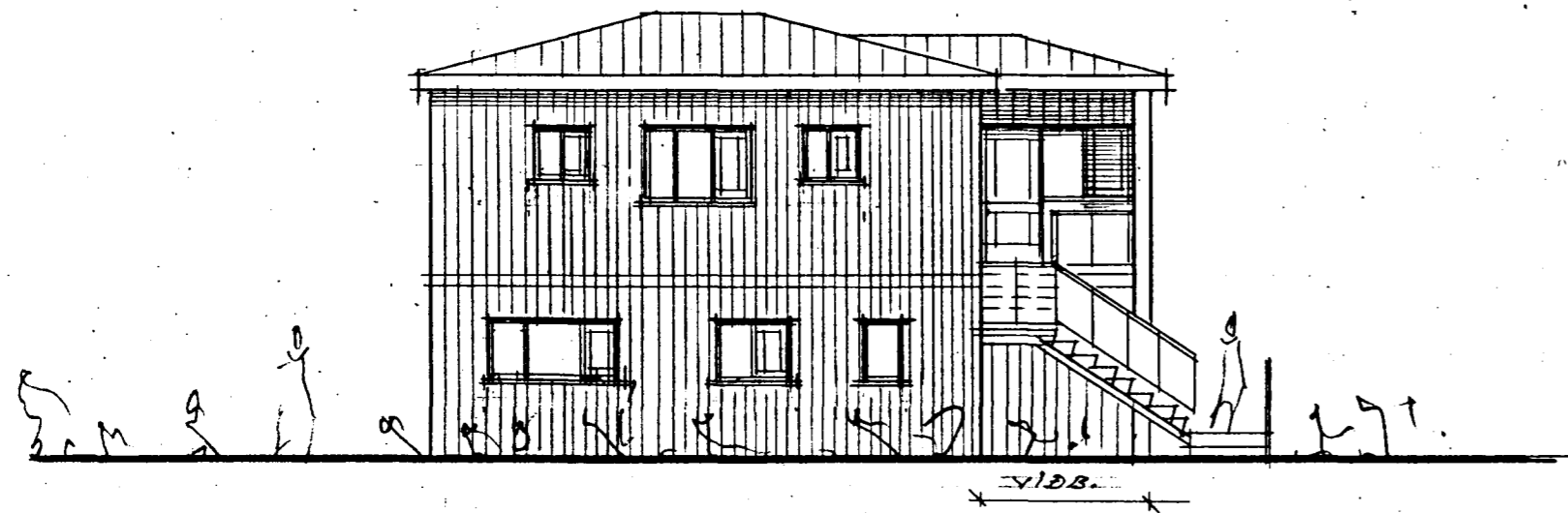
ÚTLIT AUSTUR H=1:100
