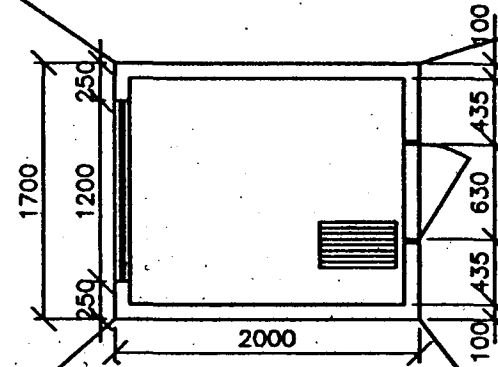
GRUNNMYND 1:50
