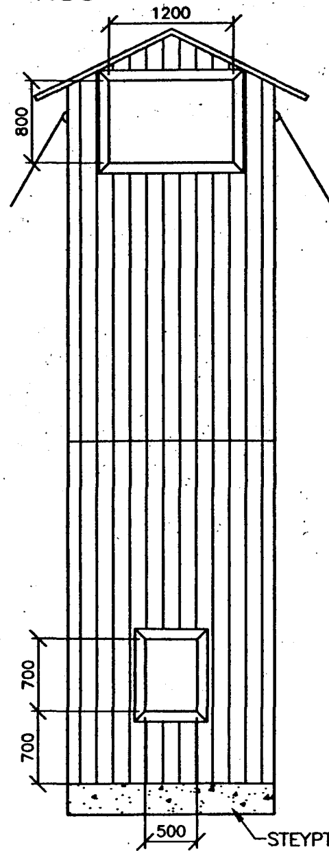
VESTURGAFL 1:50
