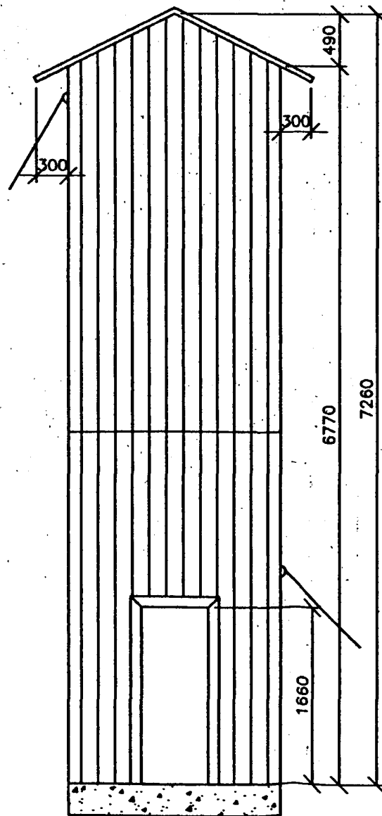
AUSTURGAFL 1:50
