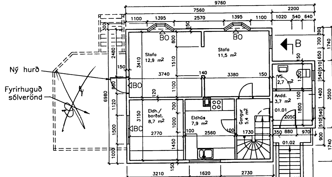
1. hæð 1:100
