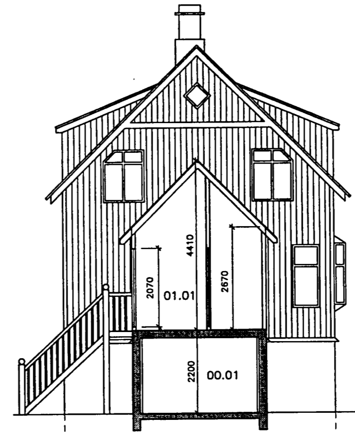
Snið B-B 1:100
