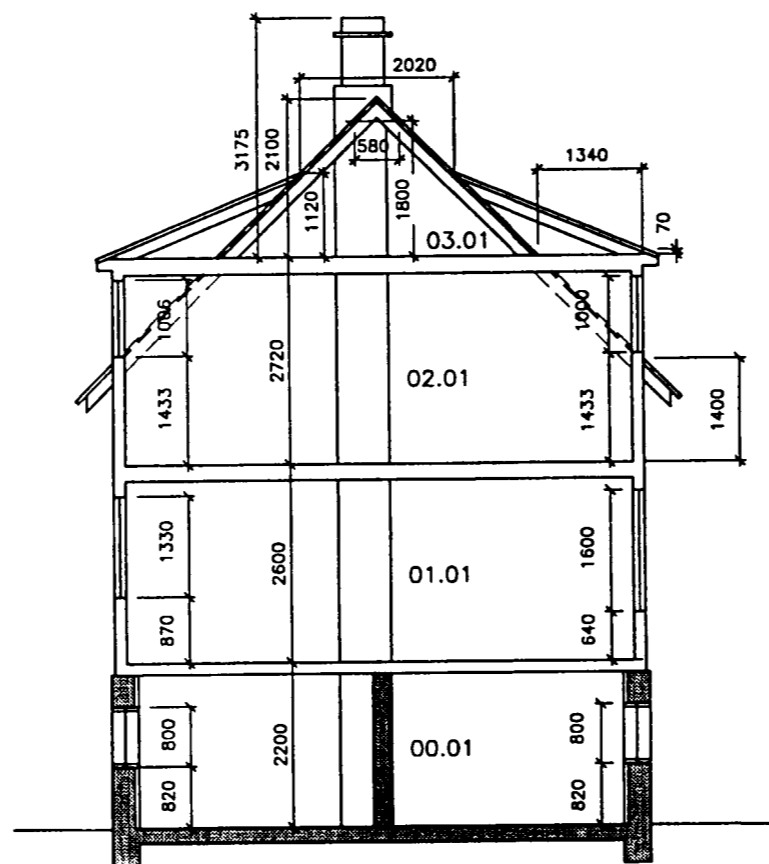
Snið A-A 1:100
