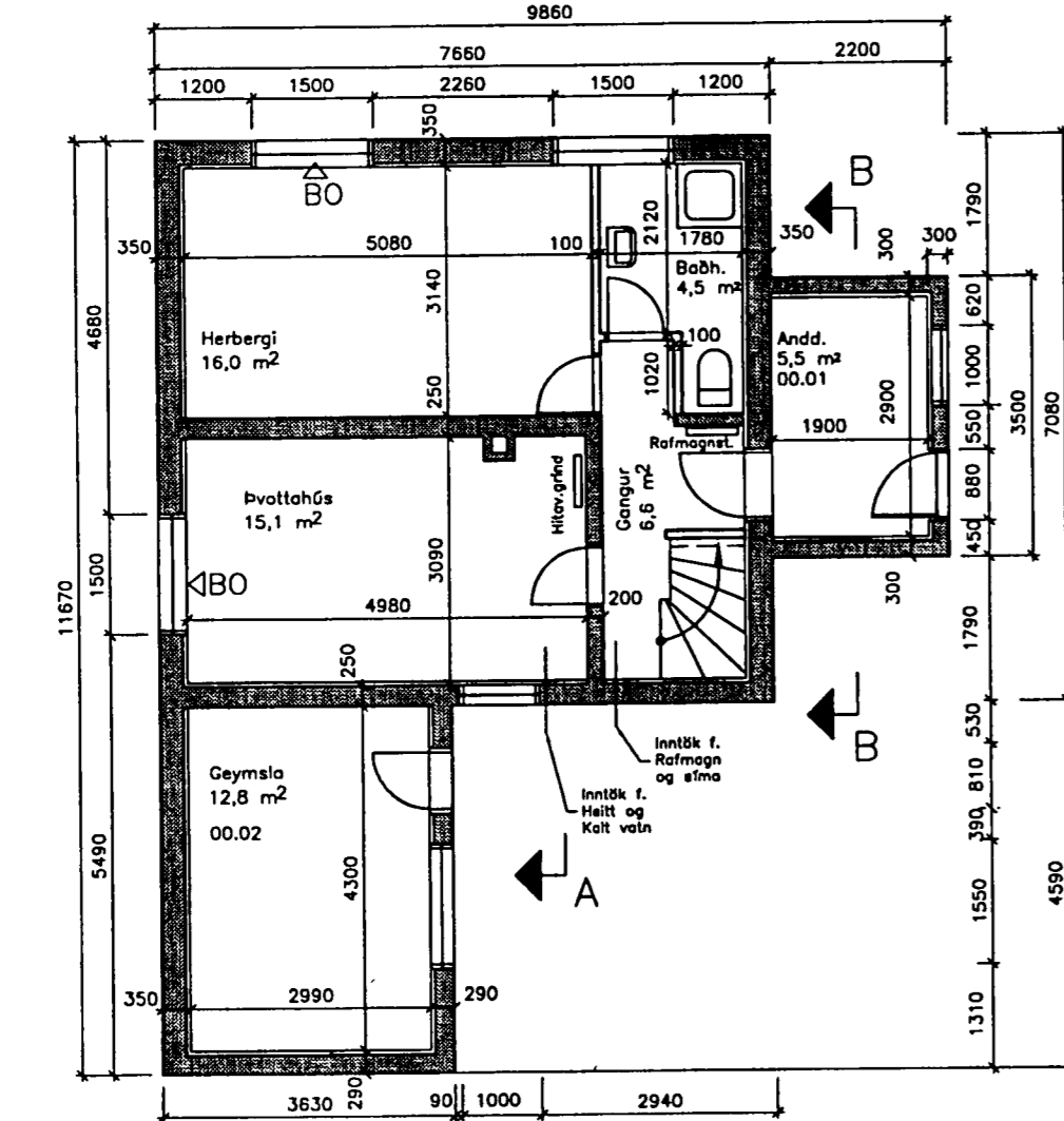
Kjallari 1:100
