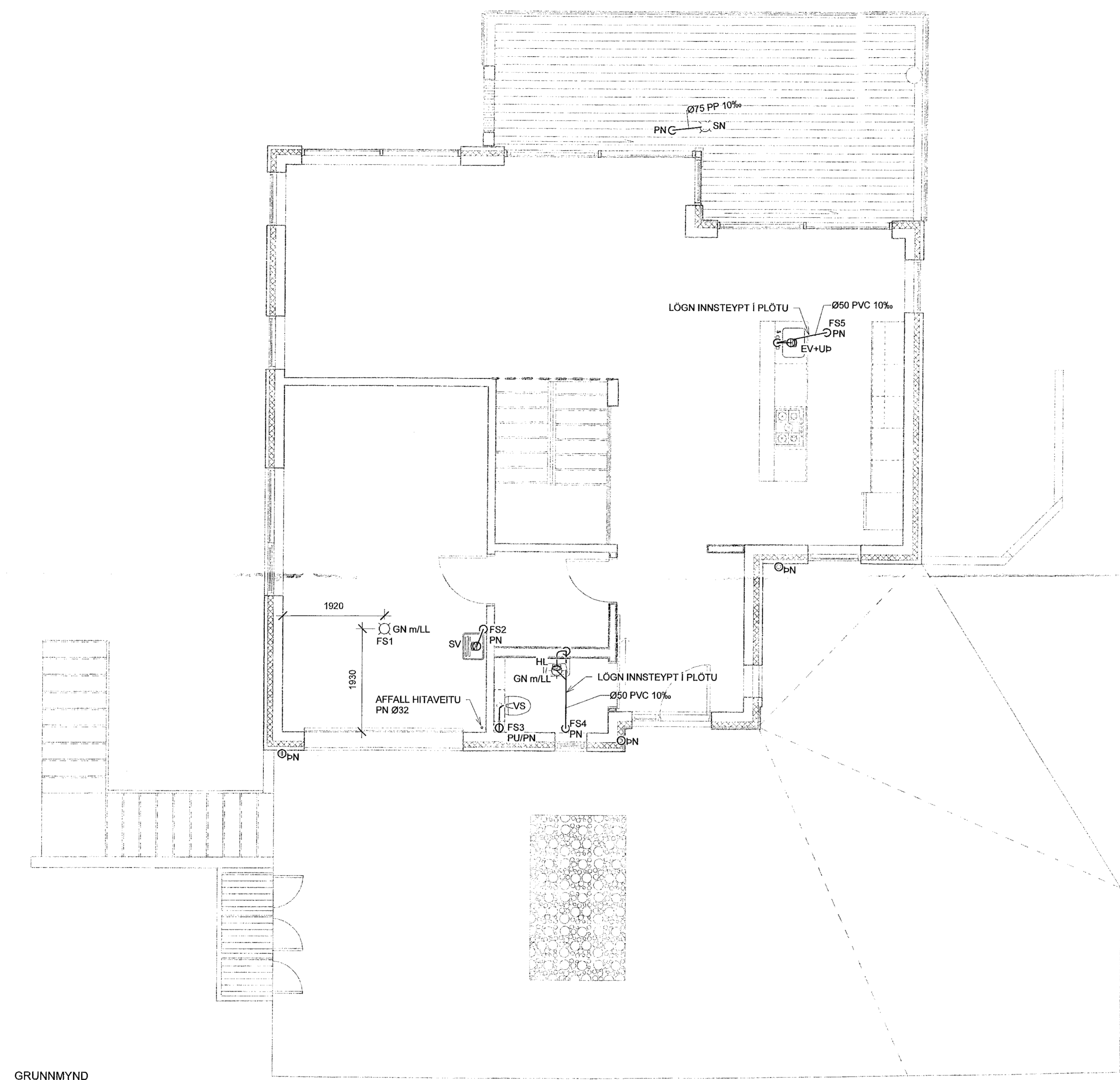
GRUNNMYND MKV. 1:50
