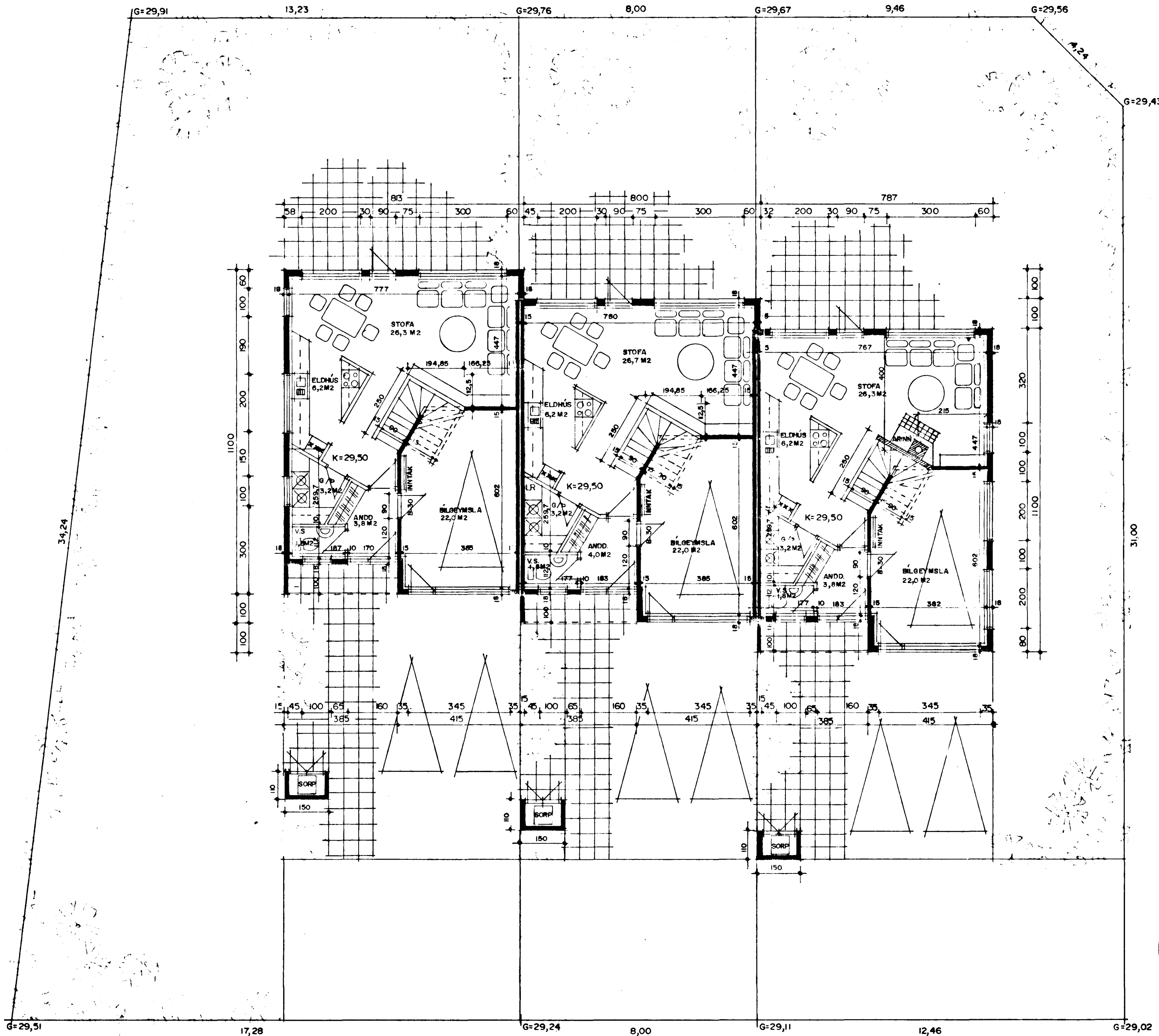
GRUNNMYND I.HÆÐ M.1:100
