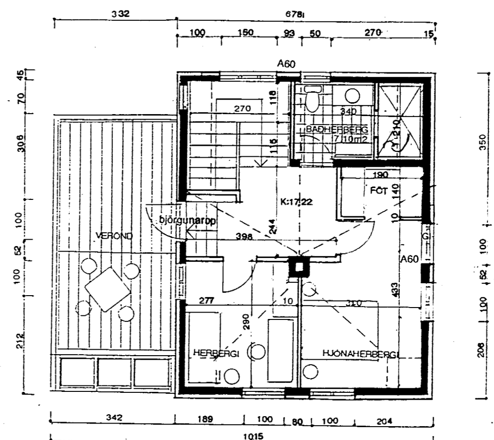
GRUNNMYND RIS mkv.1.100
