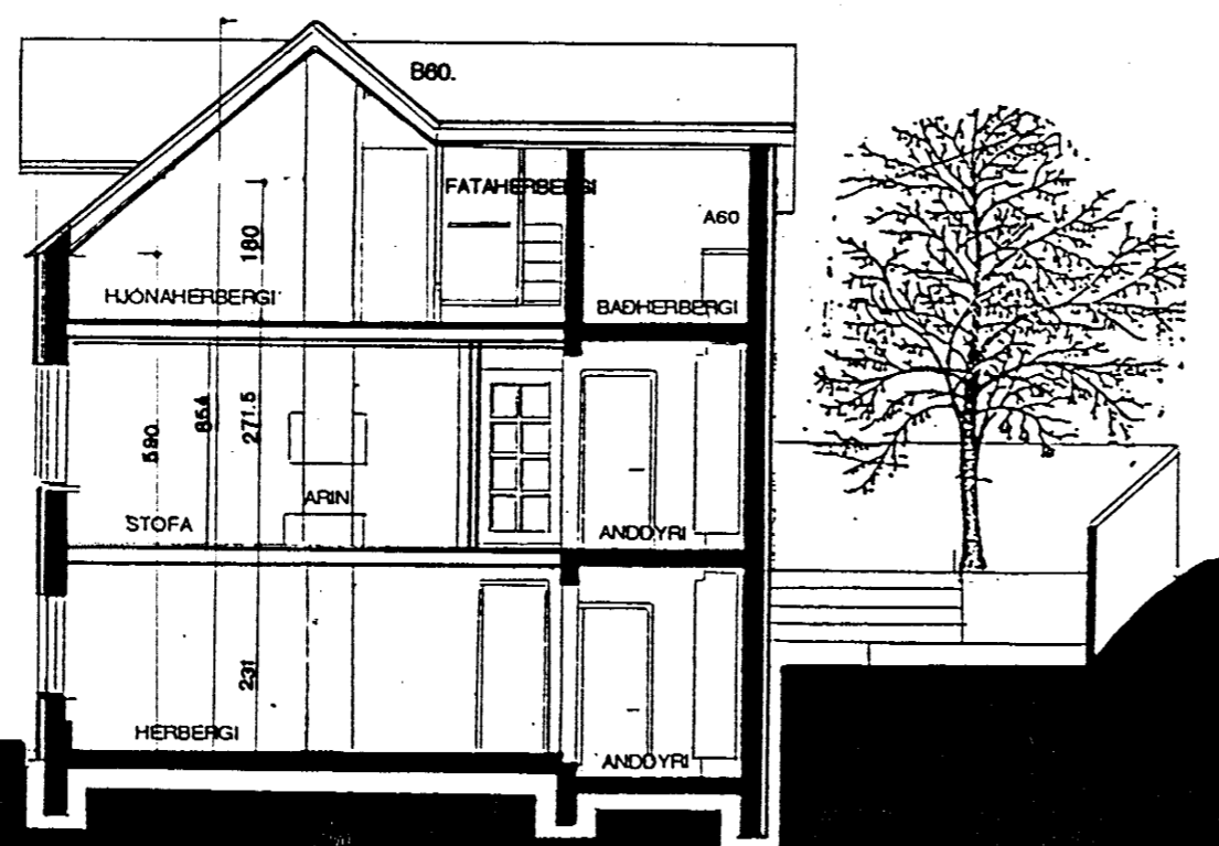
SNID A-A mkv.1.100
