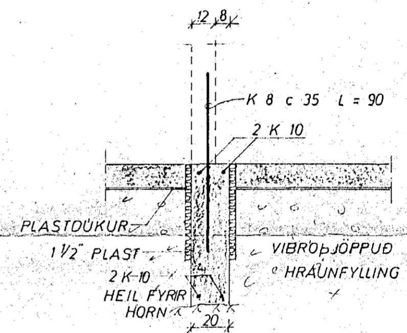
SNID 1 INNVEGG 1:20
