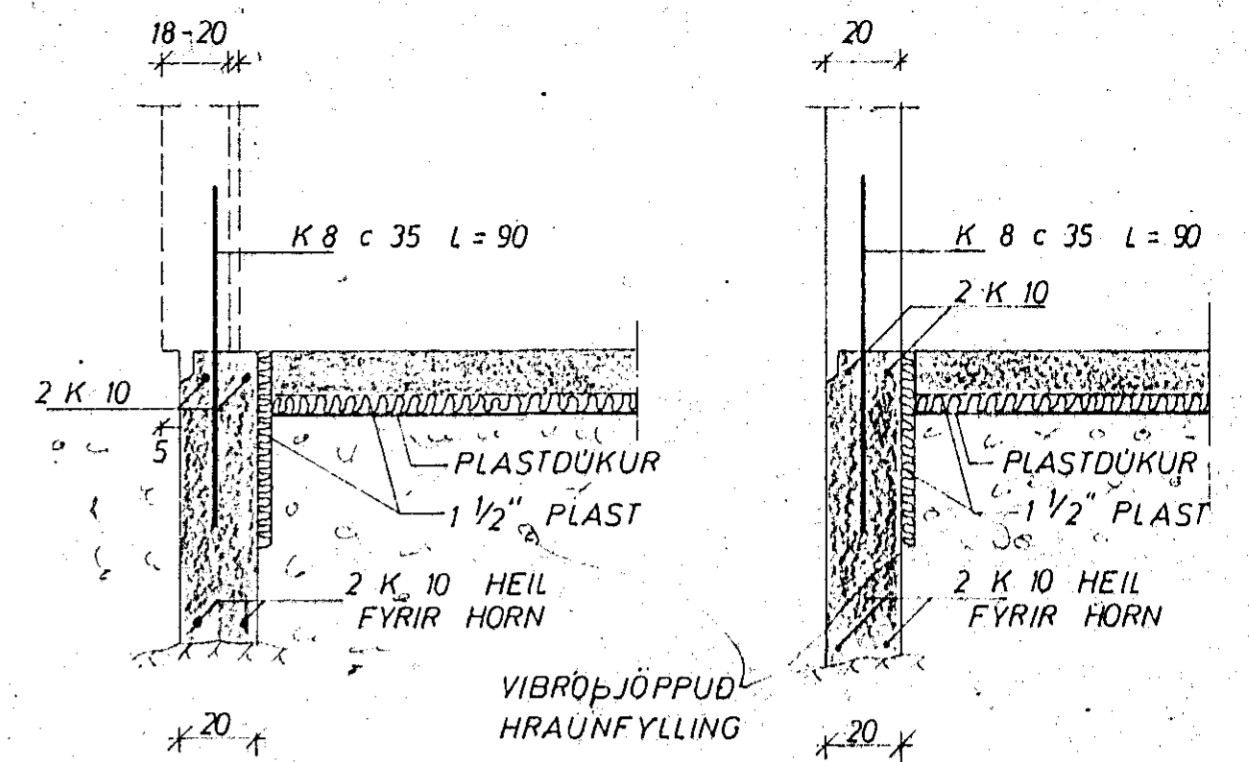
SNID 1 ÚTVEGGI 1:20
