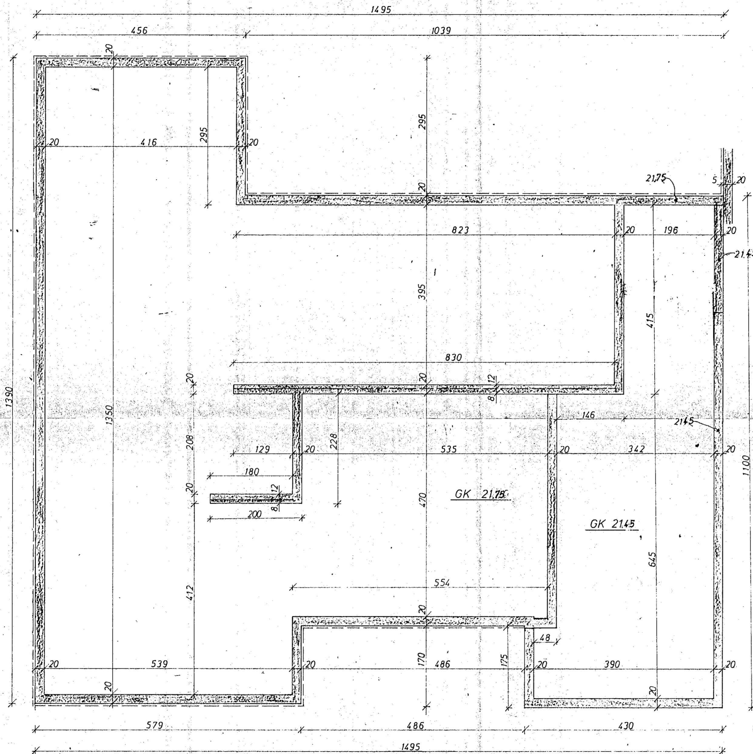
GRUNNMYND 1:50
