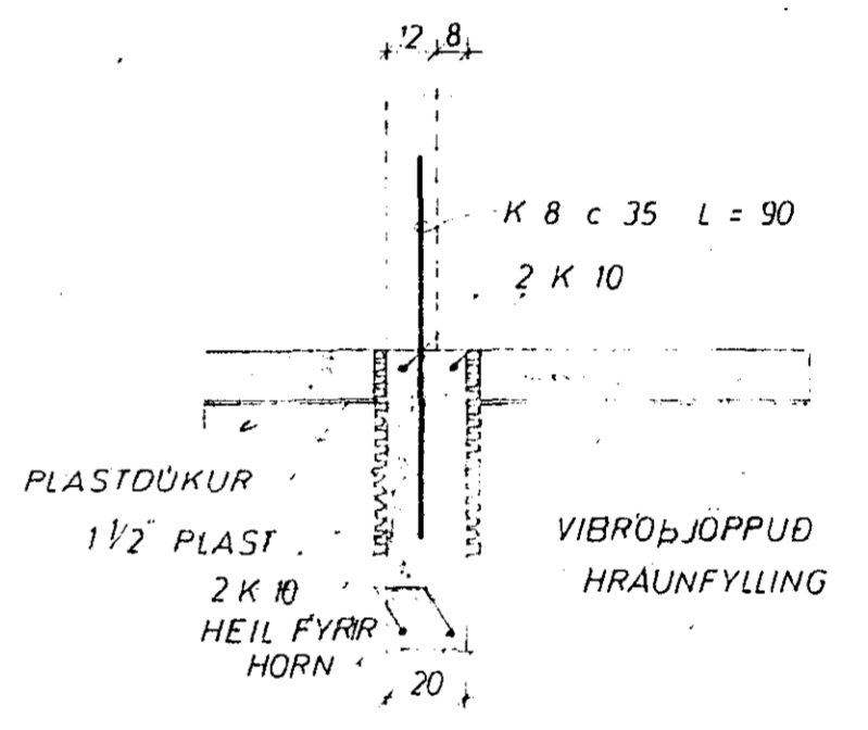
SNID 1 INNVEGG 1:20
