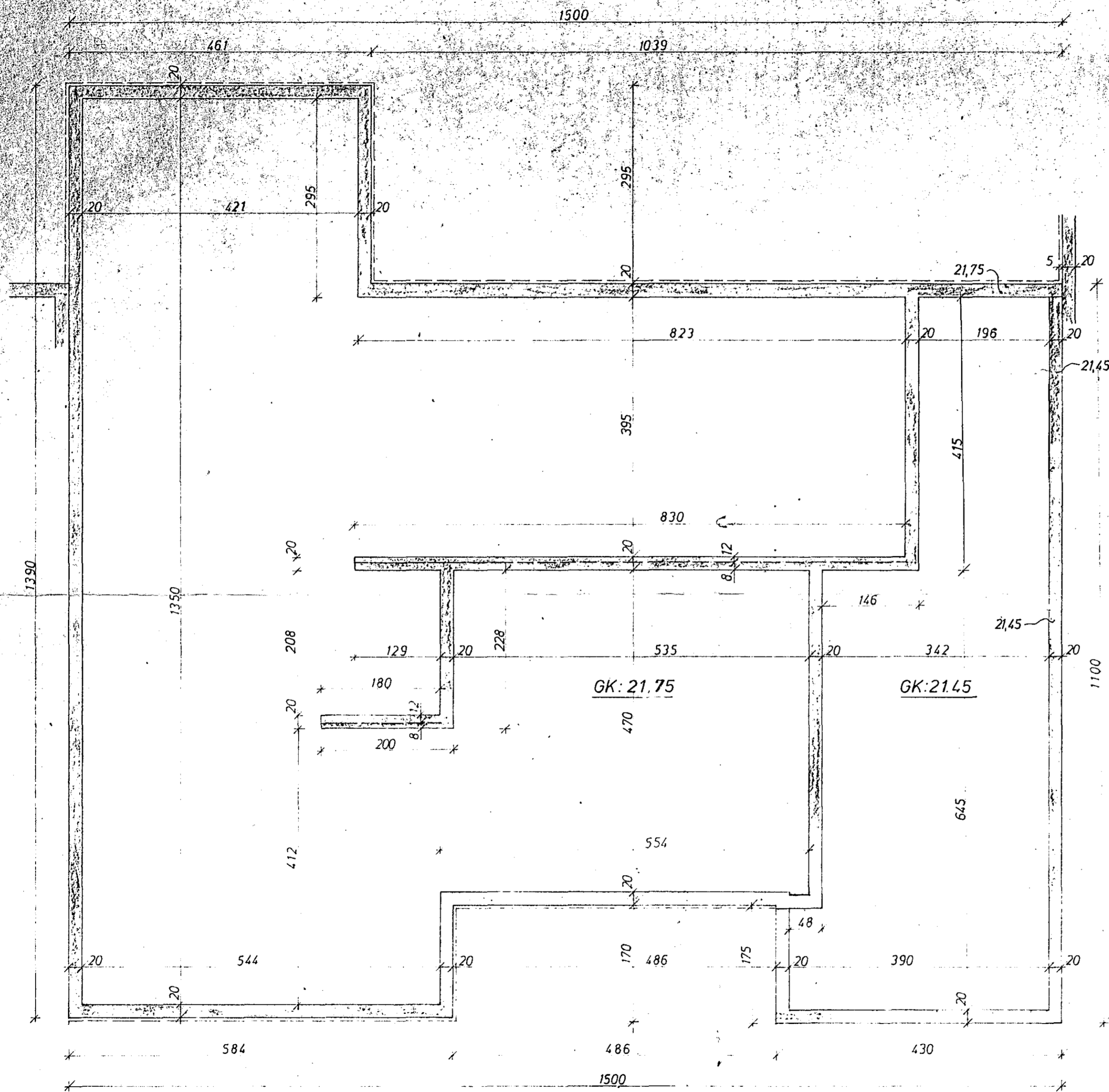
GRUNNMYND 1:50
