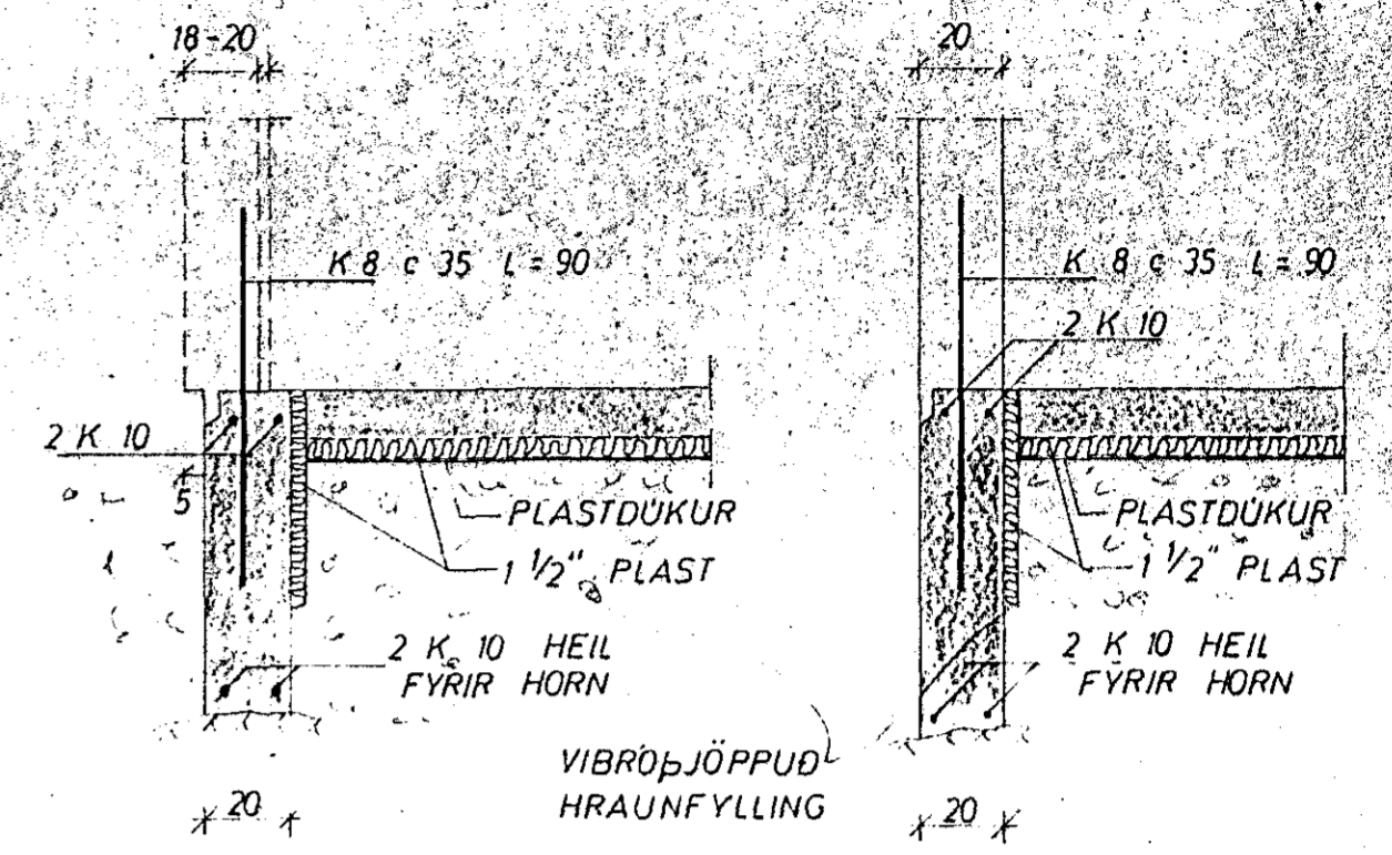
SNID 1 ÚTVEGGI 1:20
