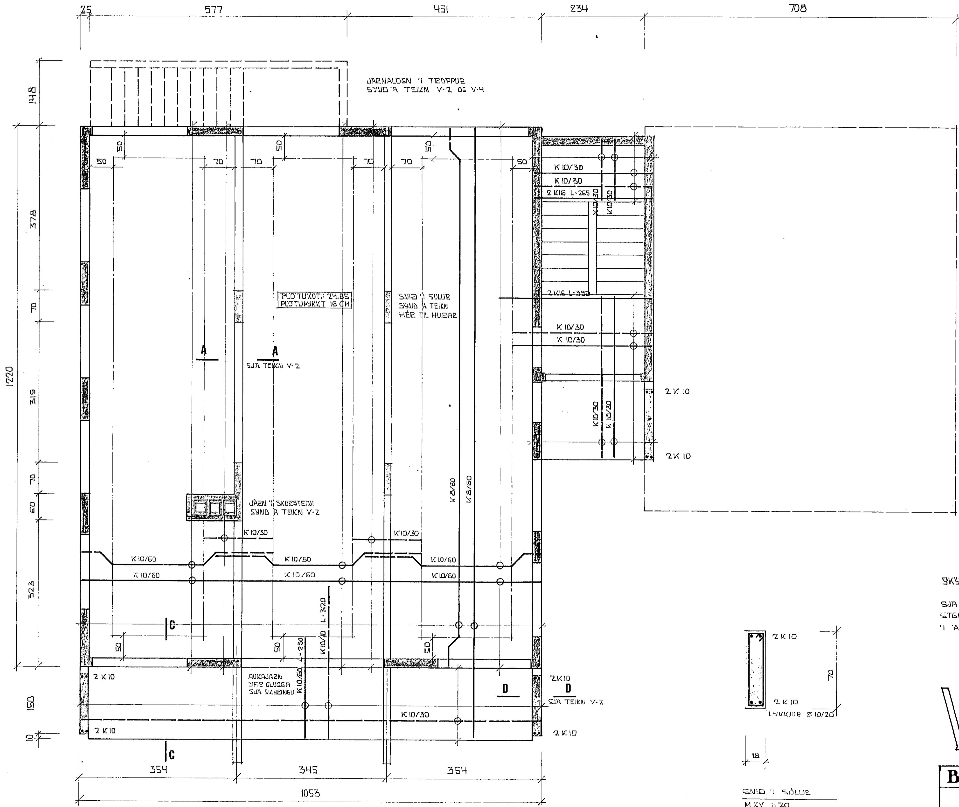
SNID I GOLFLOTTU 2 HEBAR
