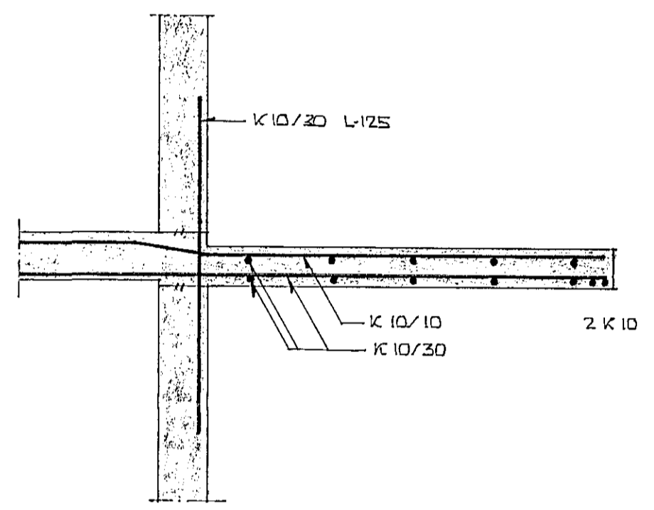
C-C SNID I SVALLIÐ MKV 1:20
