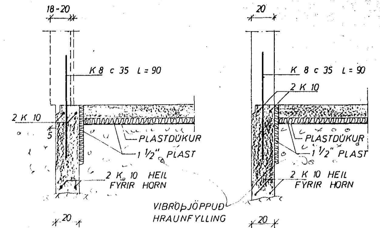
SNID 1 ÚTVEGGI 1:20
