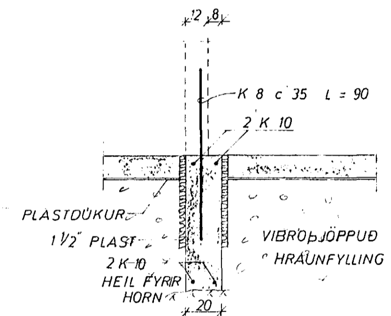
SNID 1 INNVEGG 1:20
