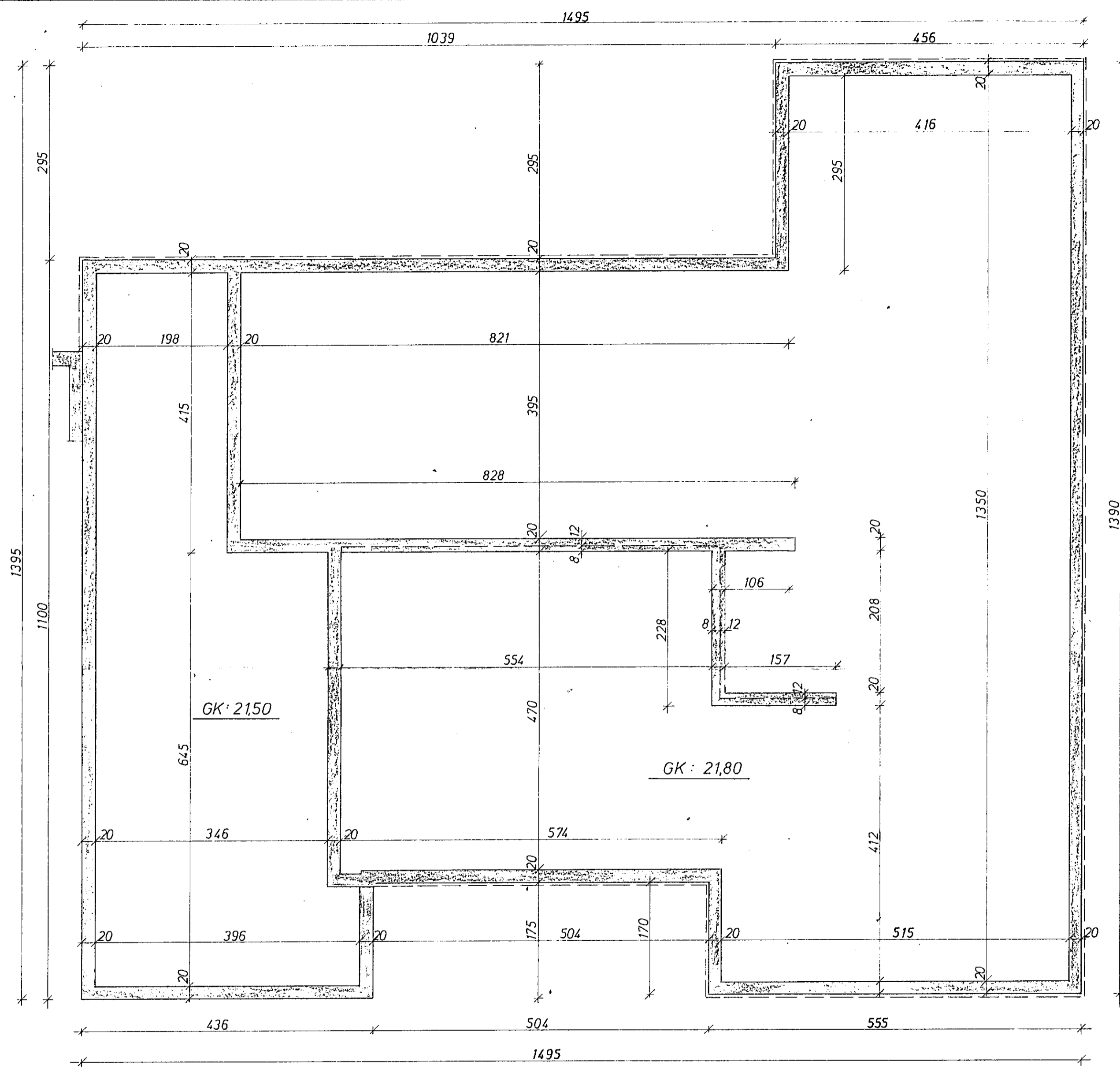
GRUNNMYND 1: 50
