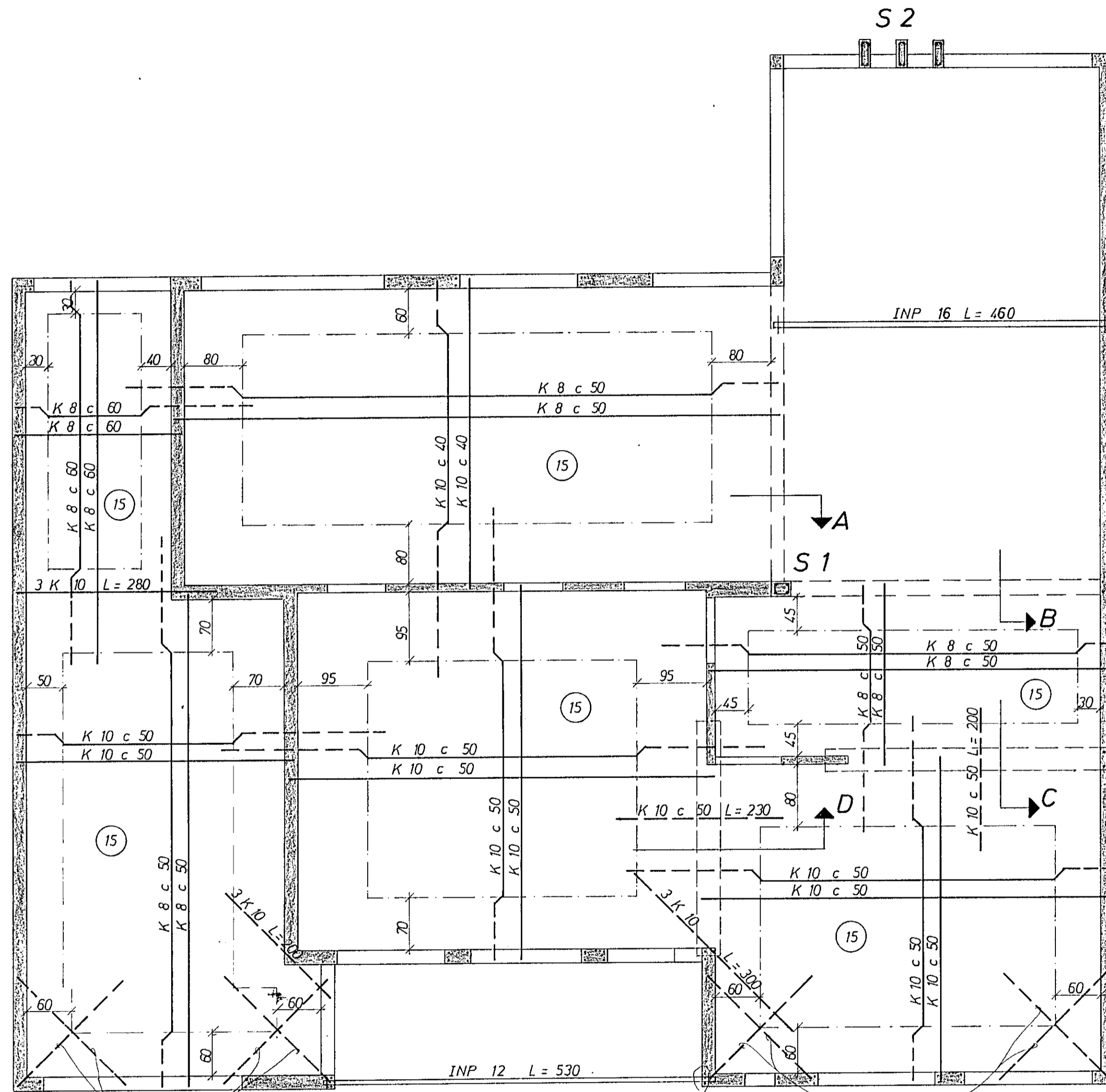
GRUNNMYND 1:50
