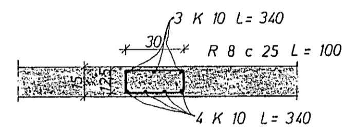
SNID D 1:20
