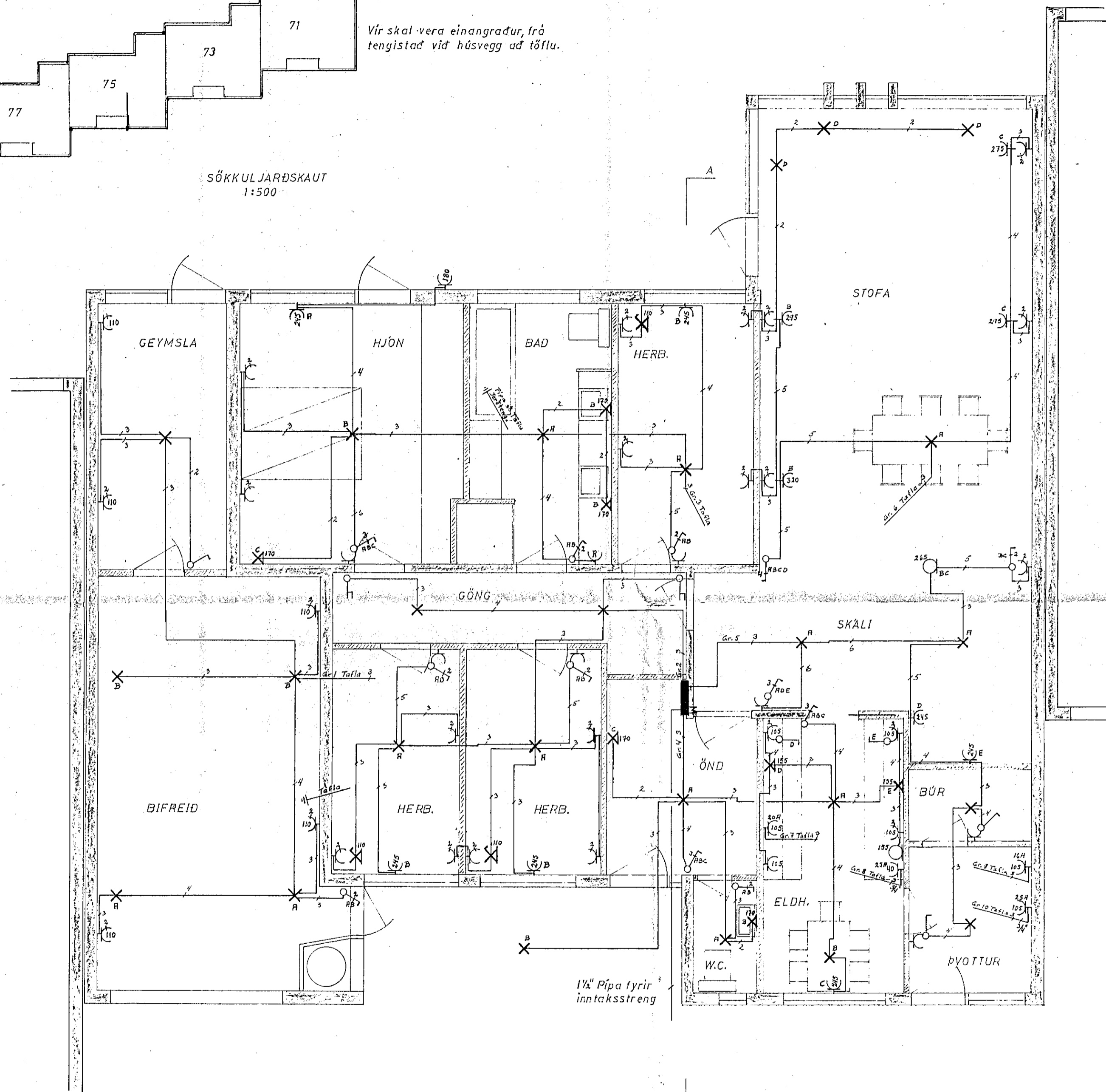
GRUNNMYND
