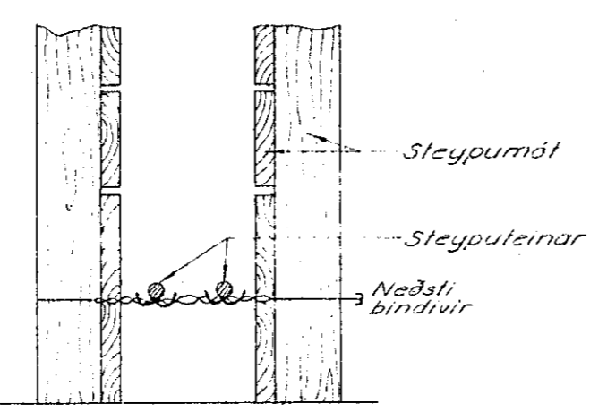
Snið í sökkul
