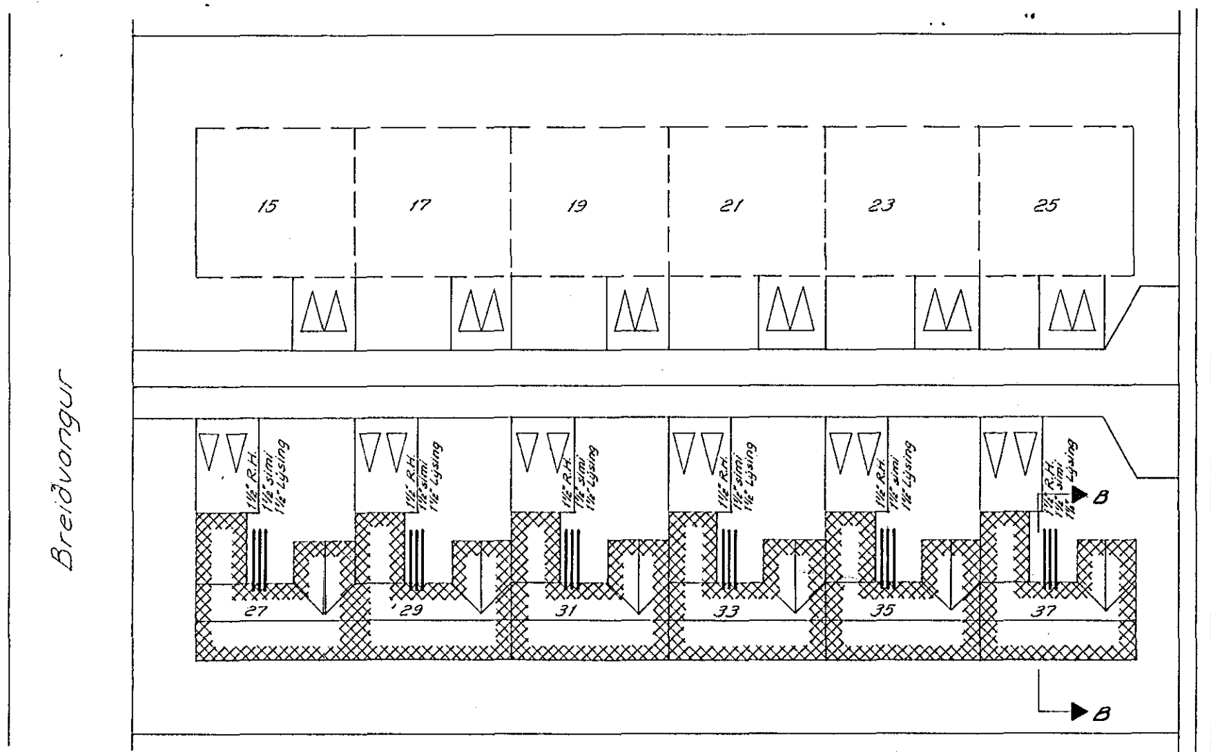
AFSTÖÐUMYND M:1:500
