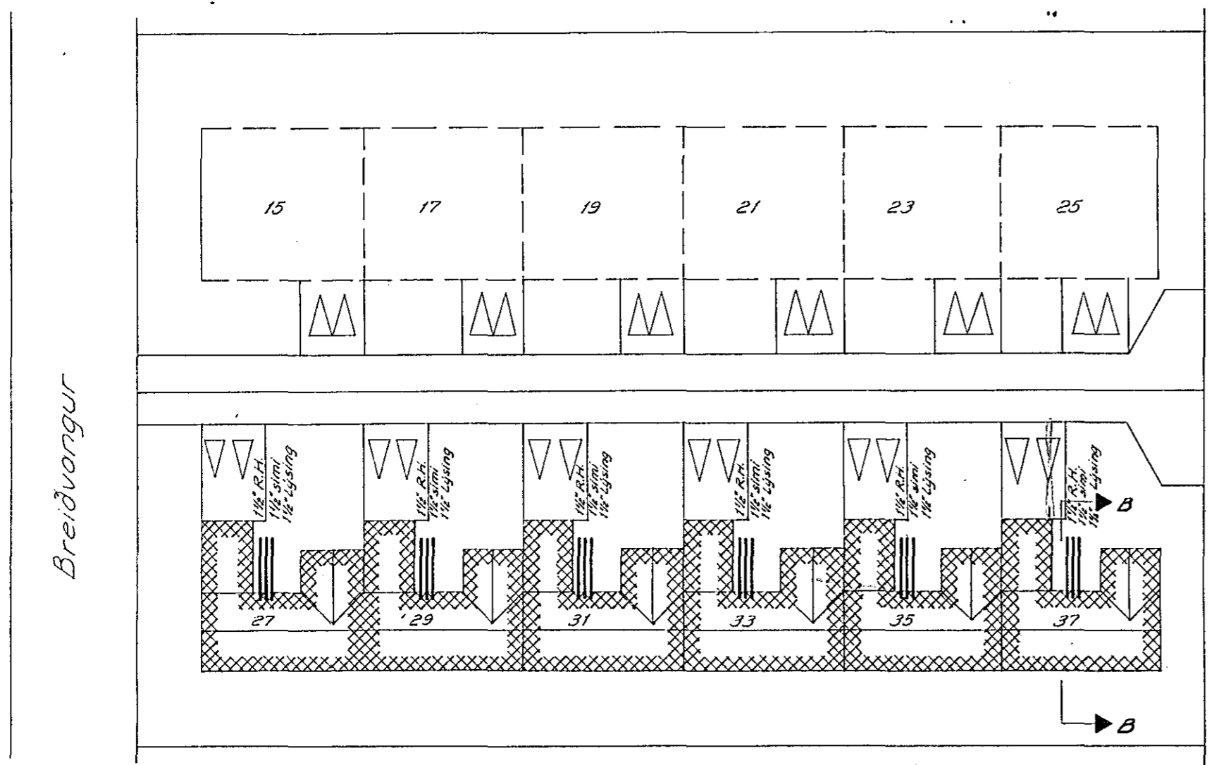
AFSTÖÐUMYND M=1:500
