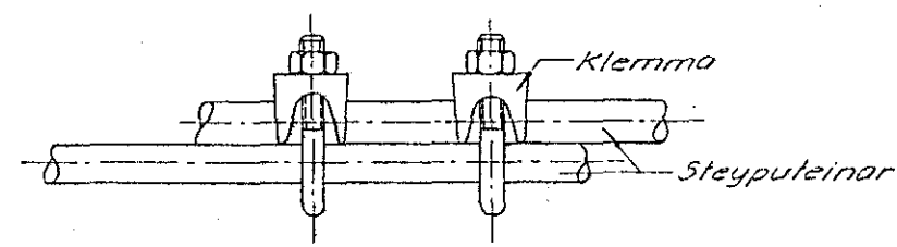
Samtenging teina allan hringinn í sökklunum
