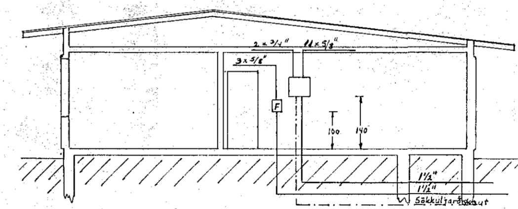
SKURÐUR A-A 1:100
