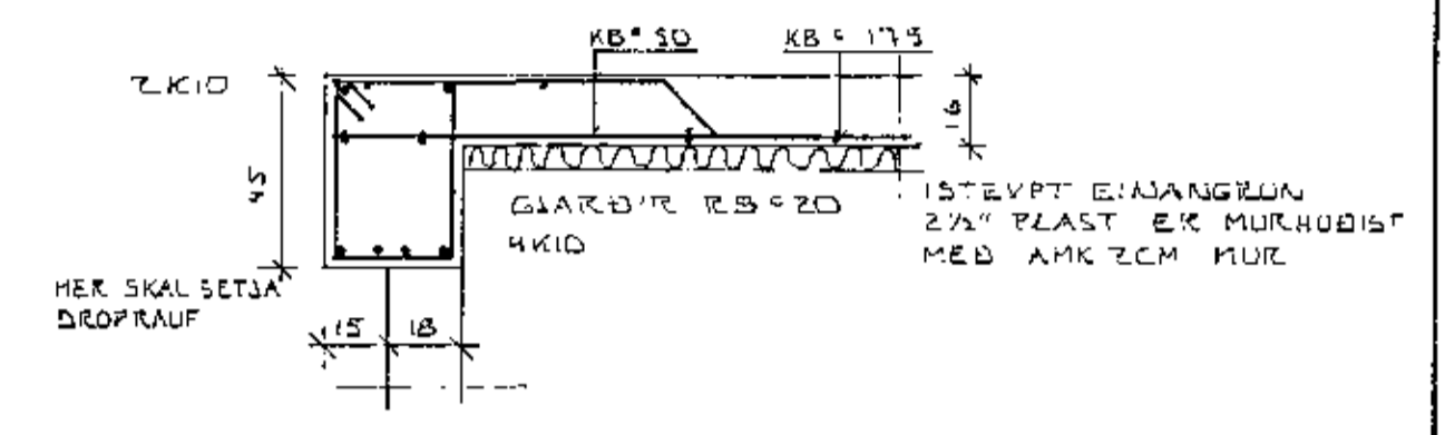
SNIÐ Í BITA YFIR DYRUM OG GLUGGA 1:20
