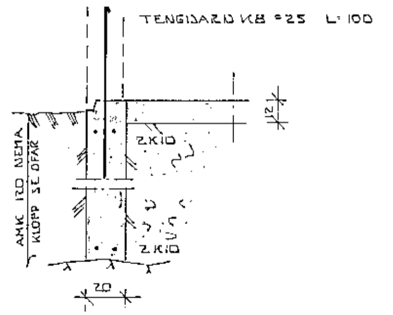
SNIÐ Í UNDIRST 1:20
