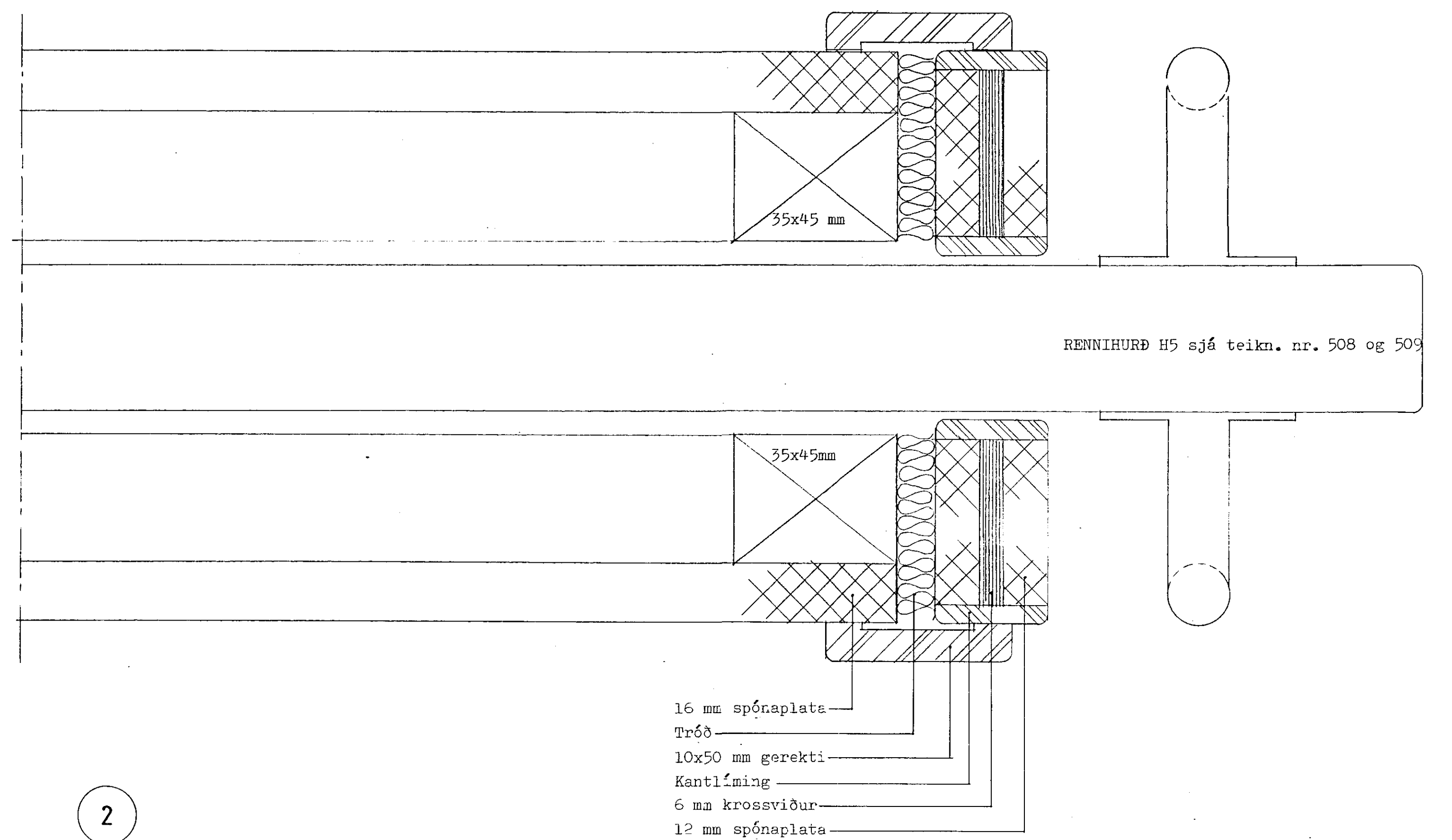
LÁRÉTT SNEIÐING Í VEGGI V1 OG V2 MEÐ RENNIHURÐ INNFELLDRI Í VEGG M 1:1
