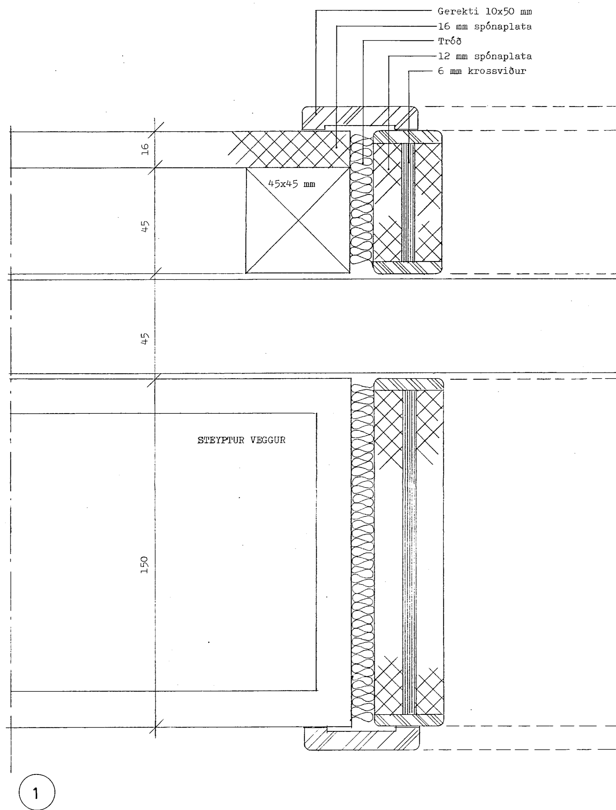
LÁRÉTT SNEIDING Í STEYPTAN VEGG VIÐ ELDHÚS MED INNBYGGÐRI RENNIHURÐ M 1:1
