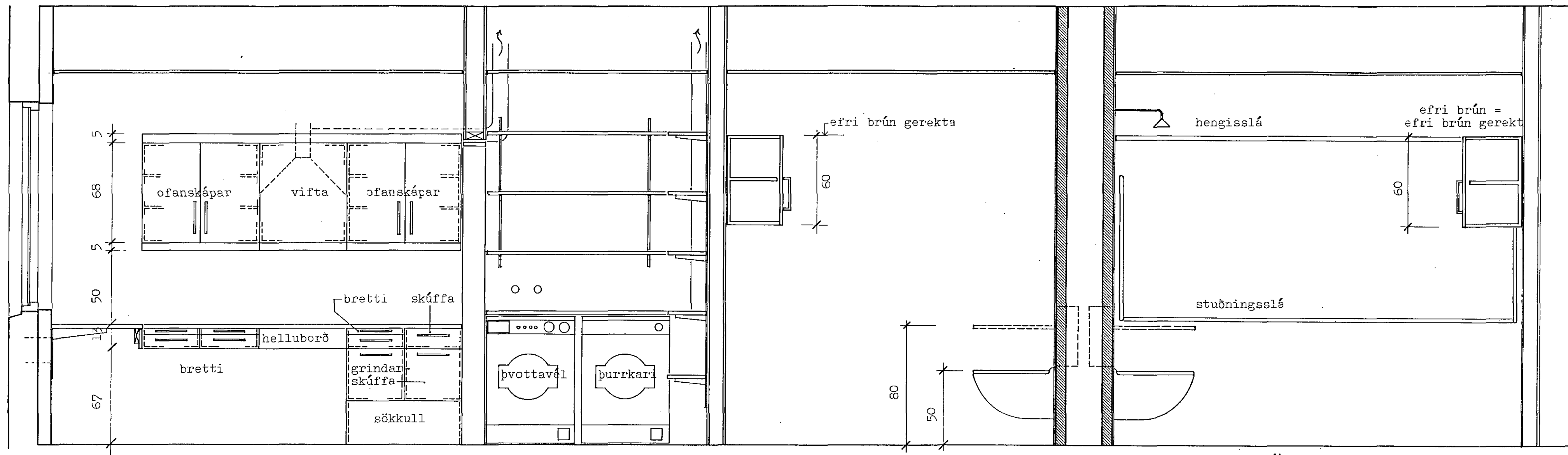
SNEIÐING A-A M 1:20
