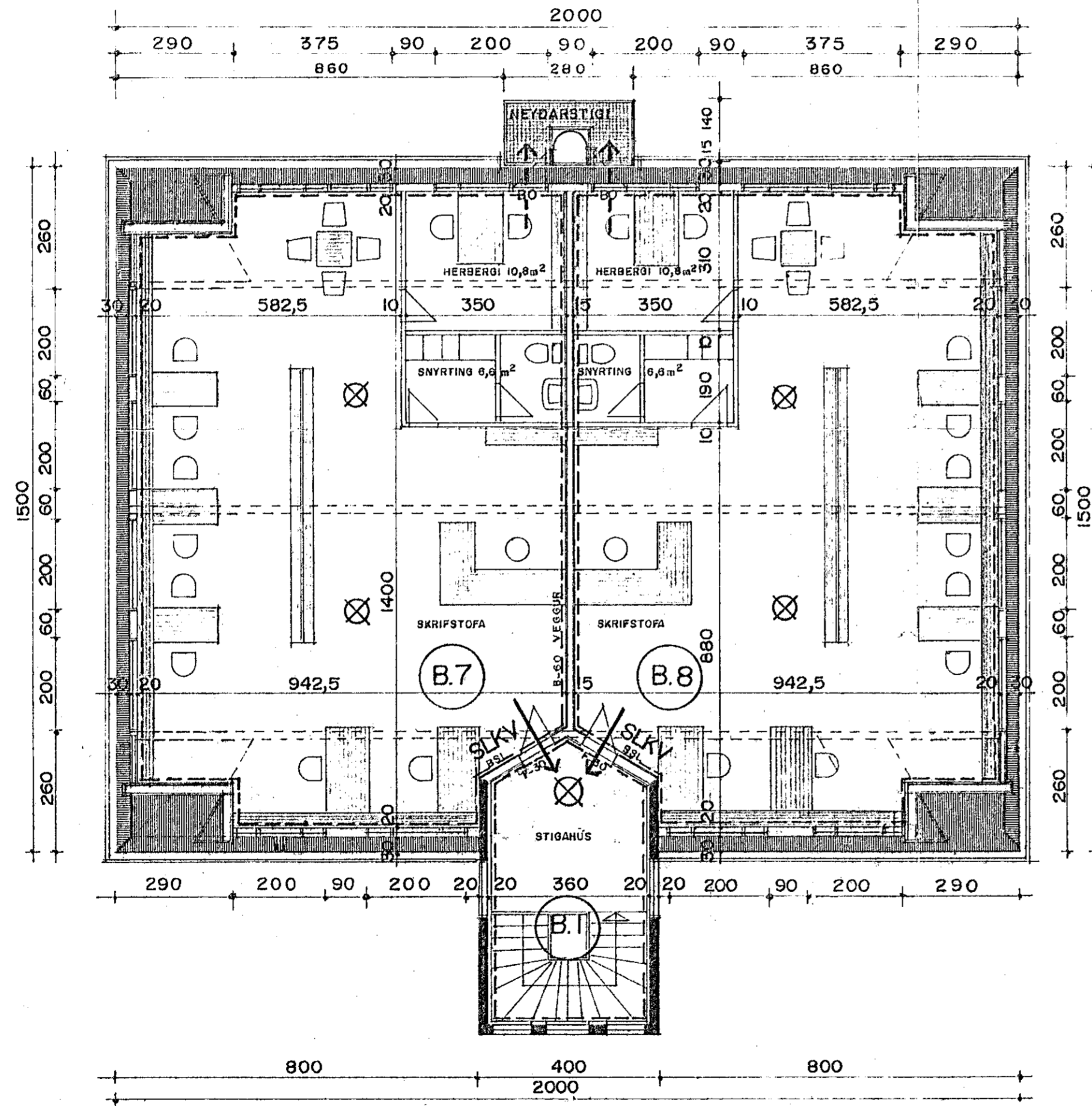
GRUNNMYND ÞAKHÆÐ M.1:100
