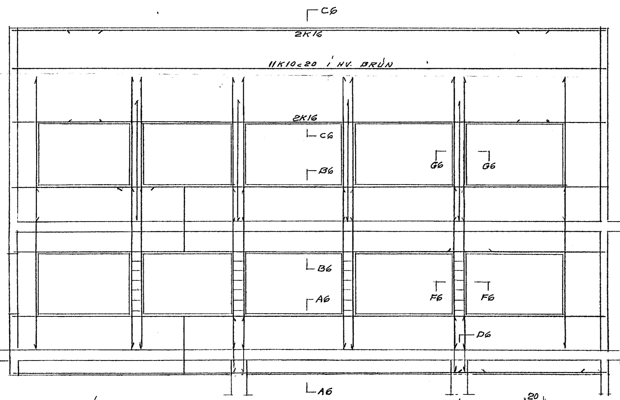
VEGGUR LÍNU D - HLUTI HLIÐARMYND 1:50
