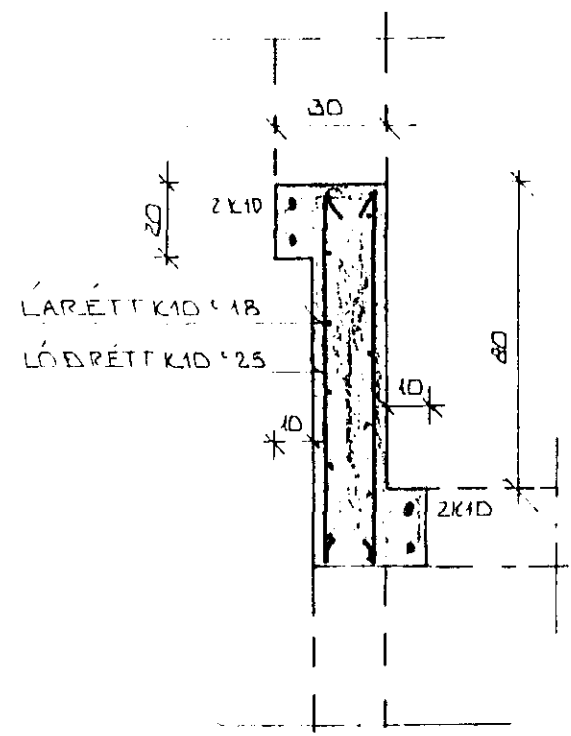
SULA S1.5. ~ 1:20
