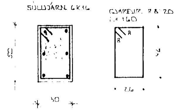
SULA S1.1. ~ 1:20
