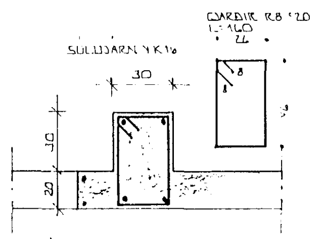
SULA S1.3. ~ 1:20
