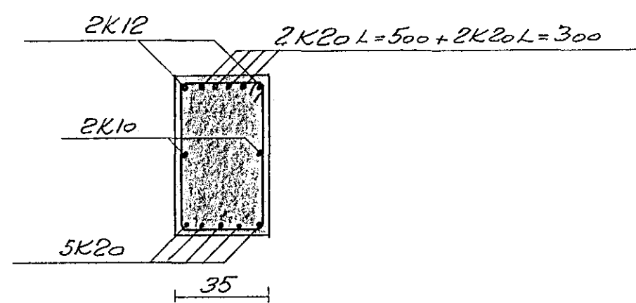
Snið B-B, 1:20
