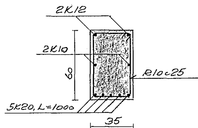
Snið A-A, 1:20
