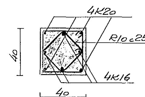
Snið D-D, 1:20
