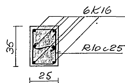
Snið E-E, 1:20
