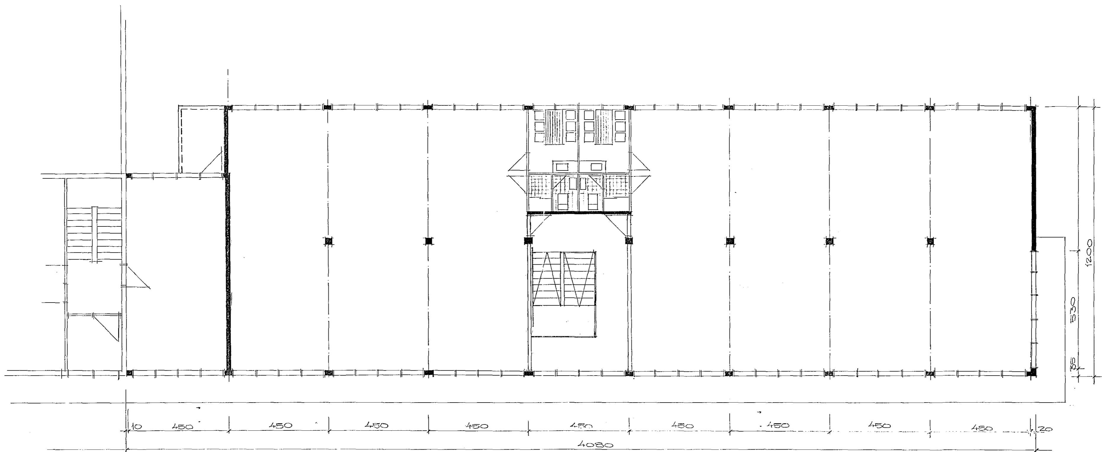
GRUNNMYND 2. HÆÐ 1:100
