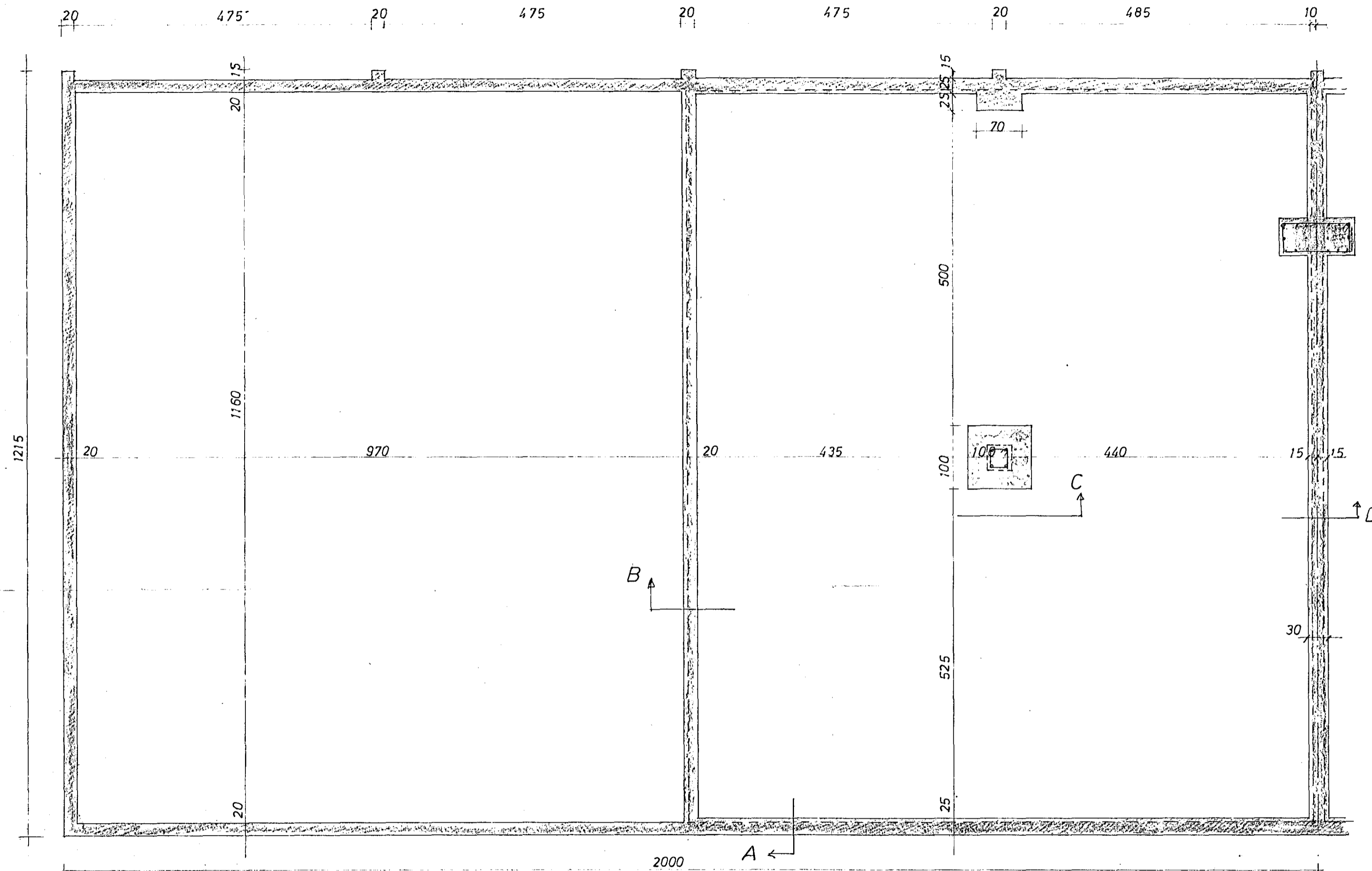
GRUNNMYND 1:50
