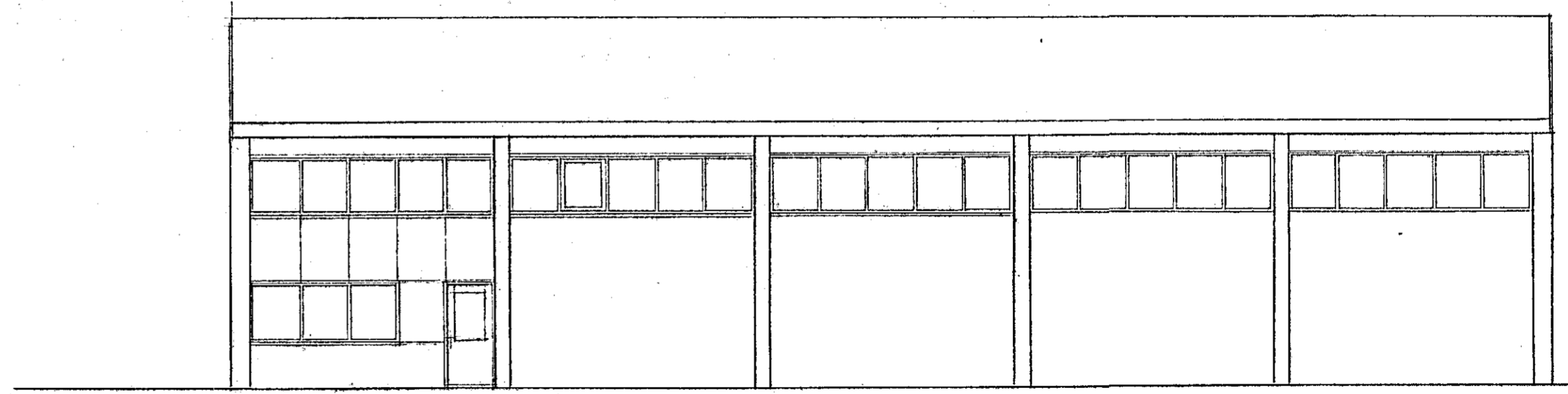
AUSTURHLID M. 1:100
