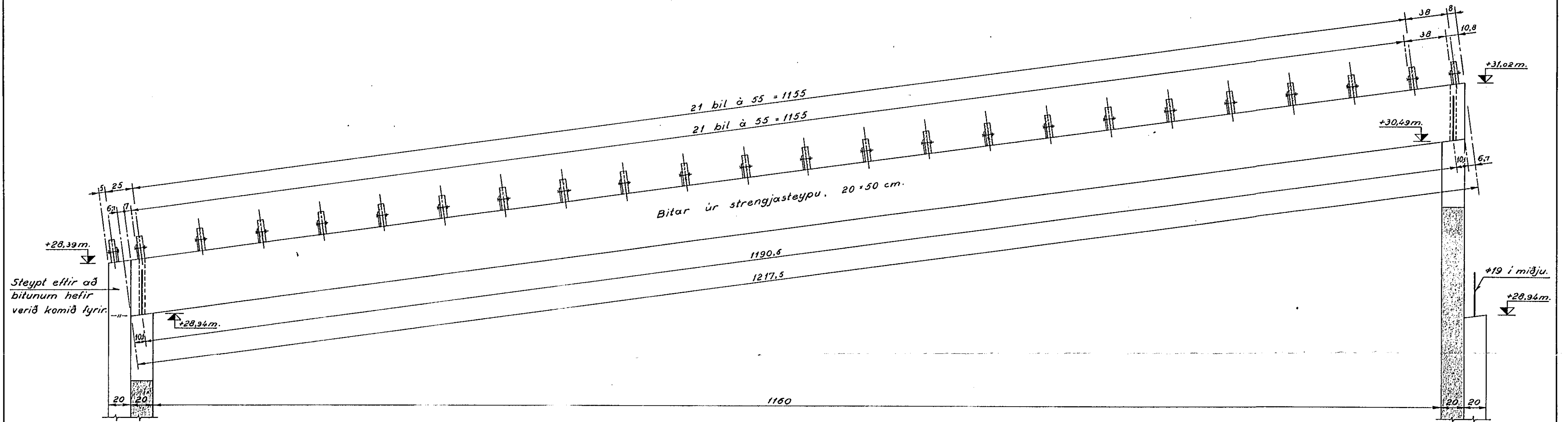
Þakbitar, 1:25.
