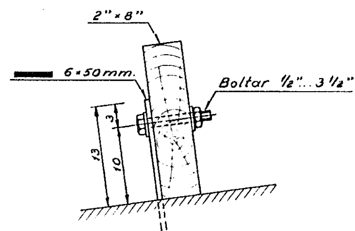
Festingar, 1:5.
