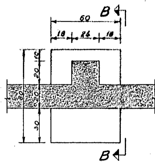
Undirstöður súlna í vesturhlíð, 1:20.
