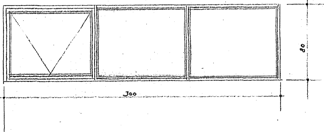
NR. 9 2 STK. HÆÐ FRÁ TILB. GÓLFI 85CM.
