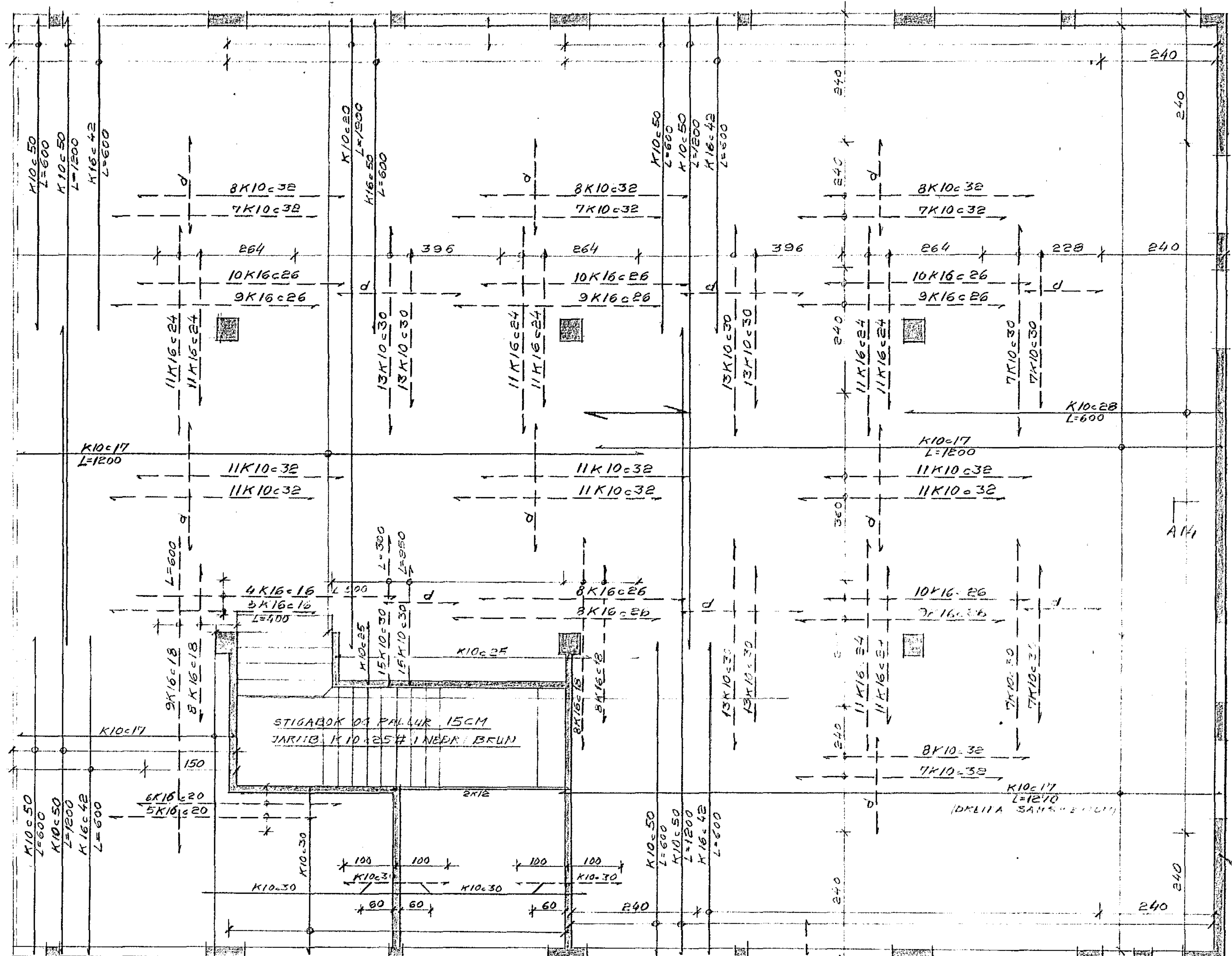
LOFT YFIR 1 HÆÐ 3. AFANGI PLÖTUR 25CM NOTPUNGI 500KG/M 2 - 1:50 -
