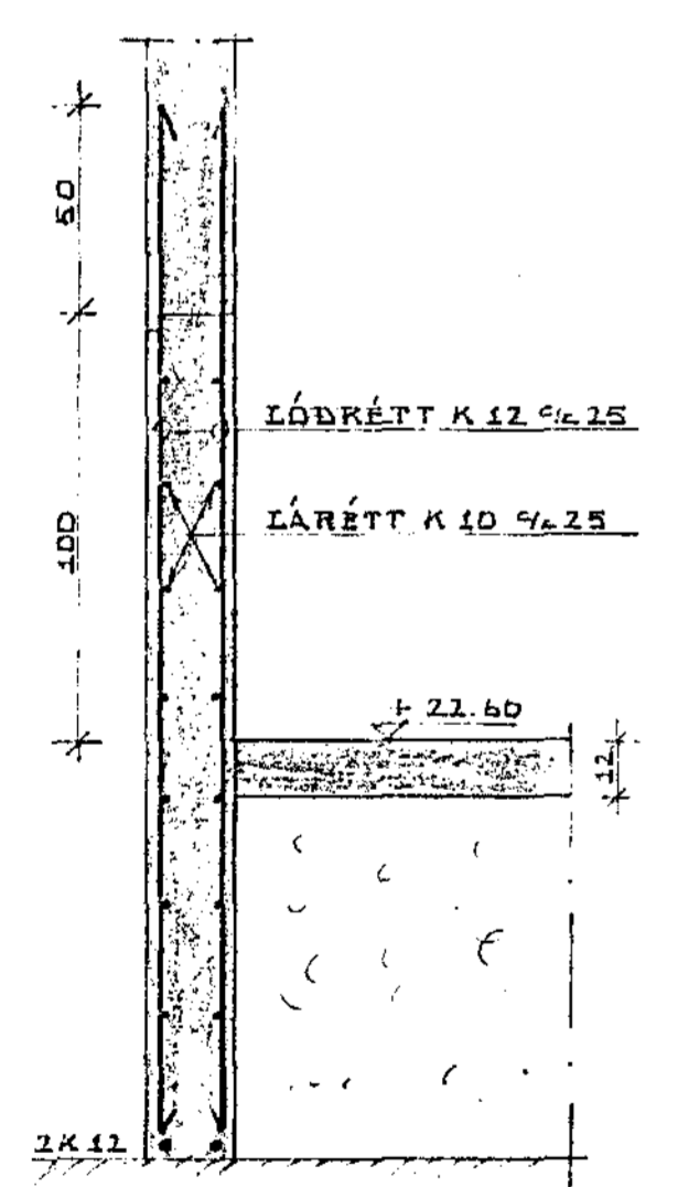
SNID A-A 1:20
