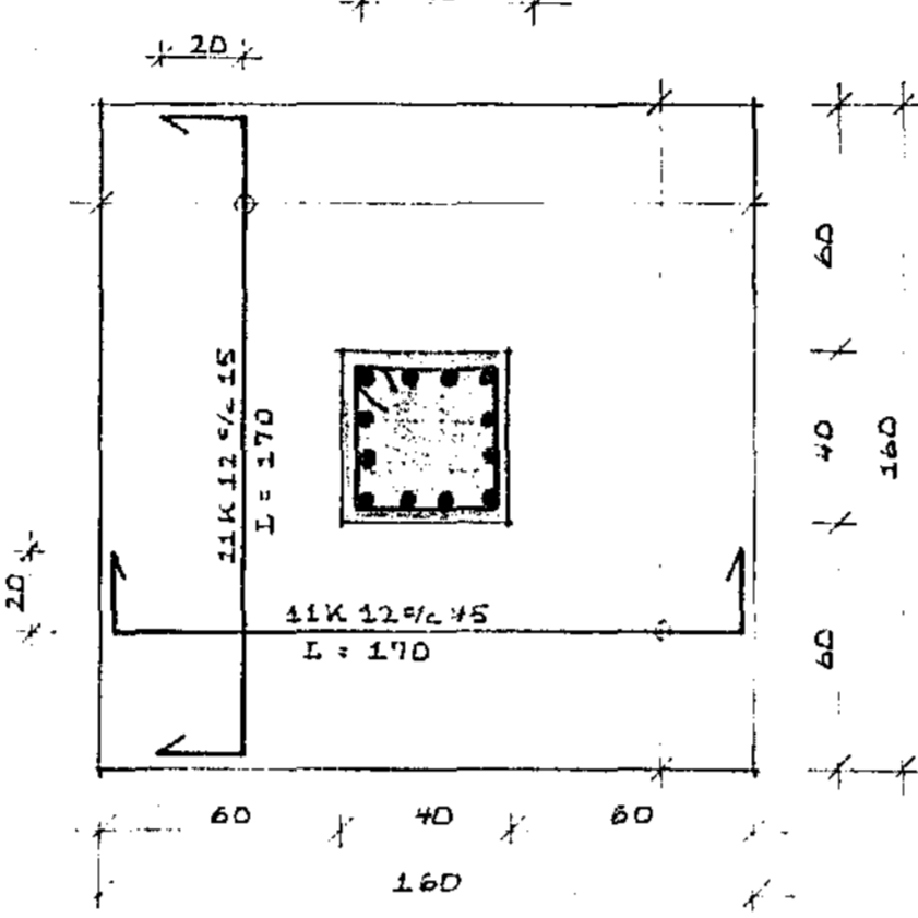
UNDIRSTADA U3 1:20
