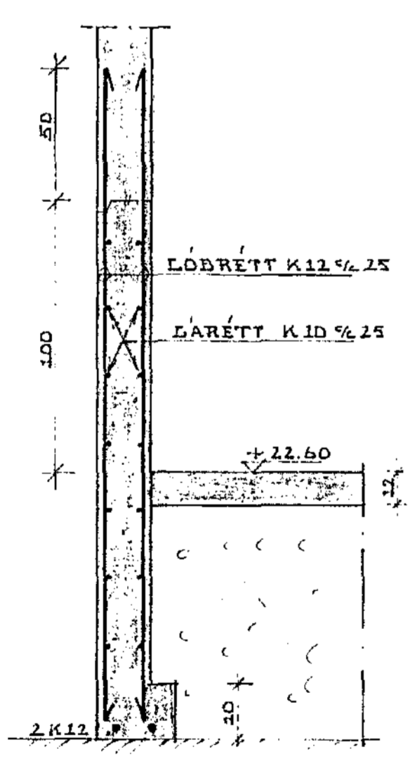
SNID B-B 1:20
