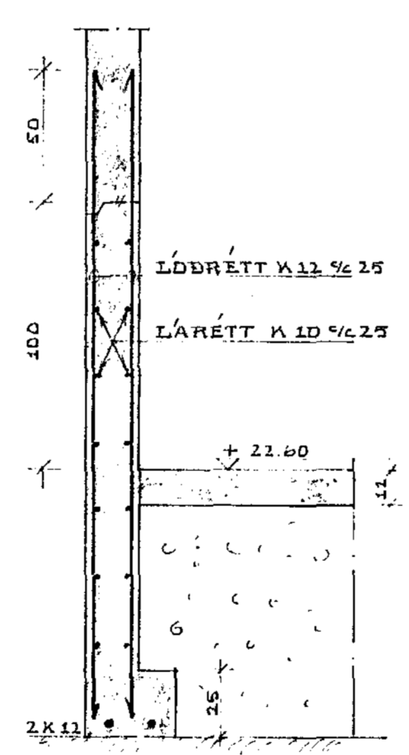
SNID D-D 1:20
