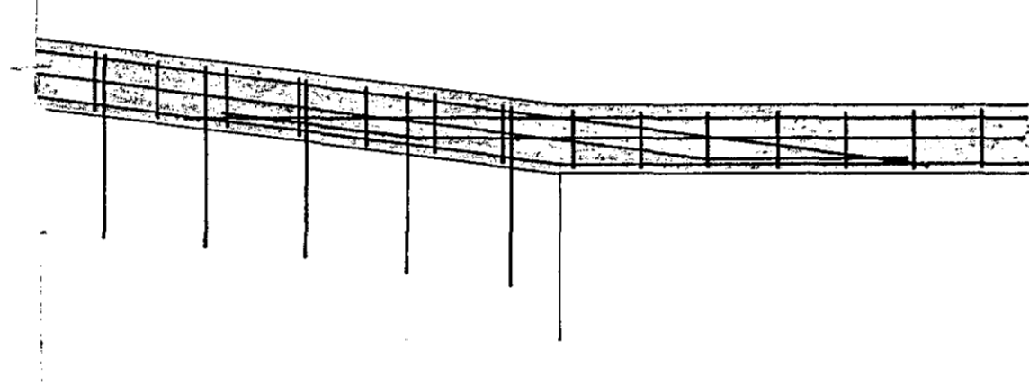
SM A SÉÐ OFAN Á BITA 1:20
