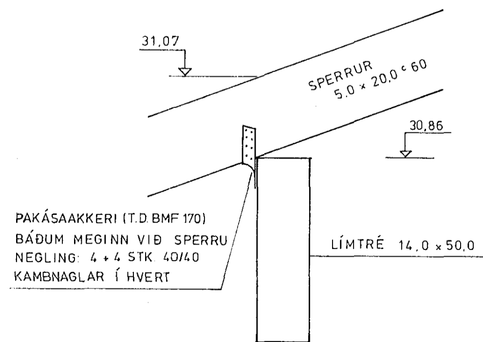
SÉRMYND D 1:10
