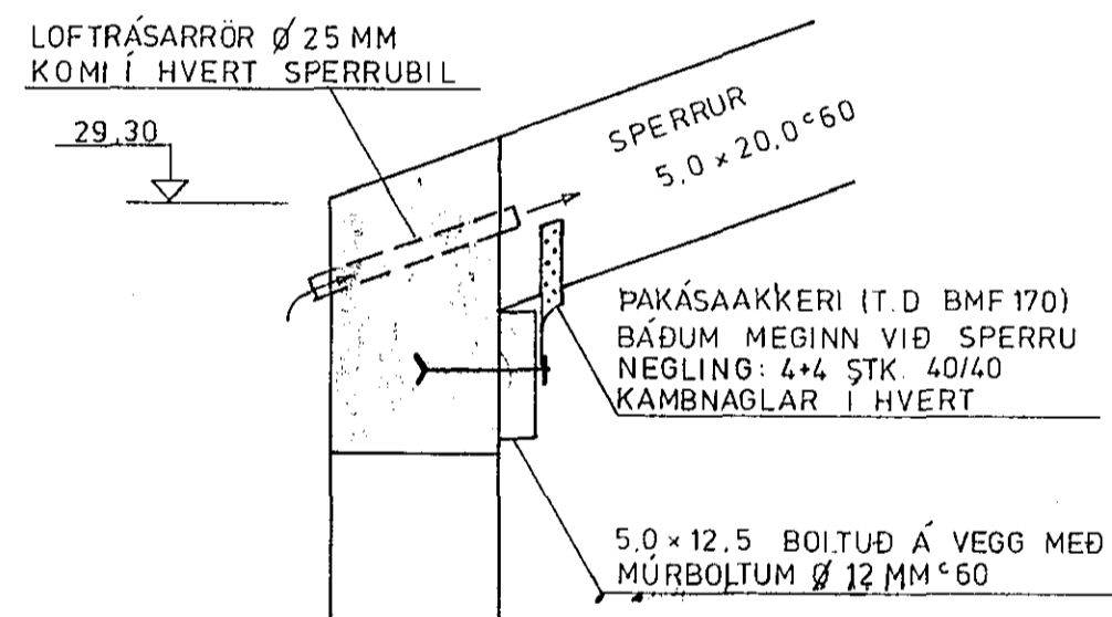
SÉRMYND A 1:10
