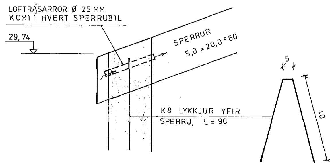
SÉRMYND B 1:10
