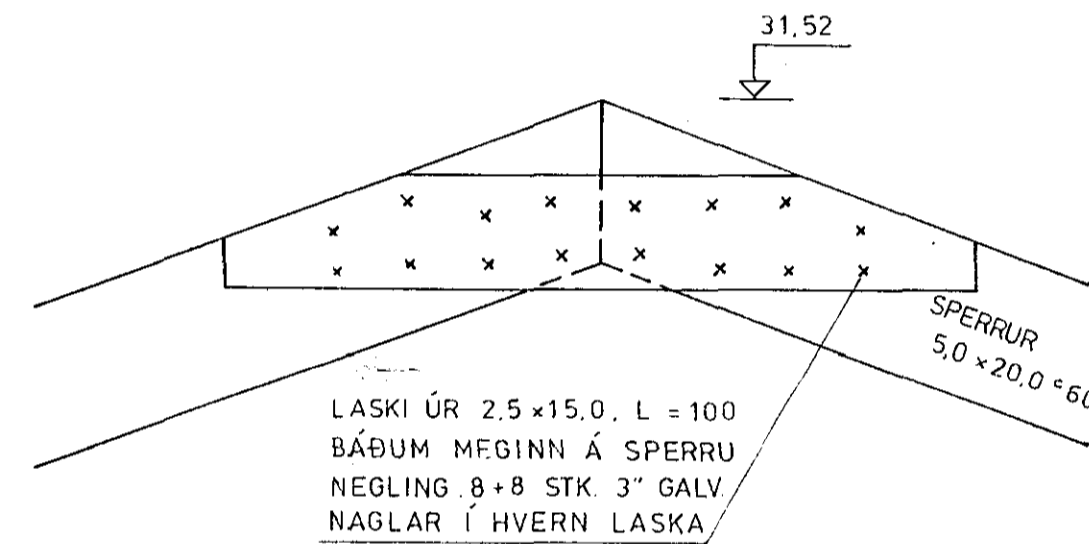
SÉRMYND C 1:10
