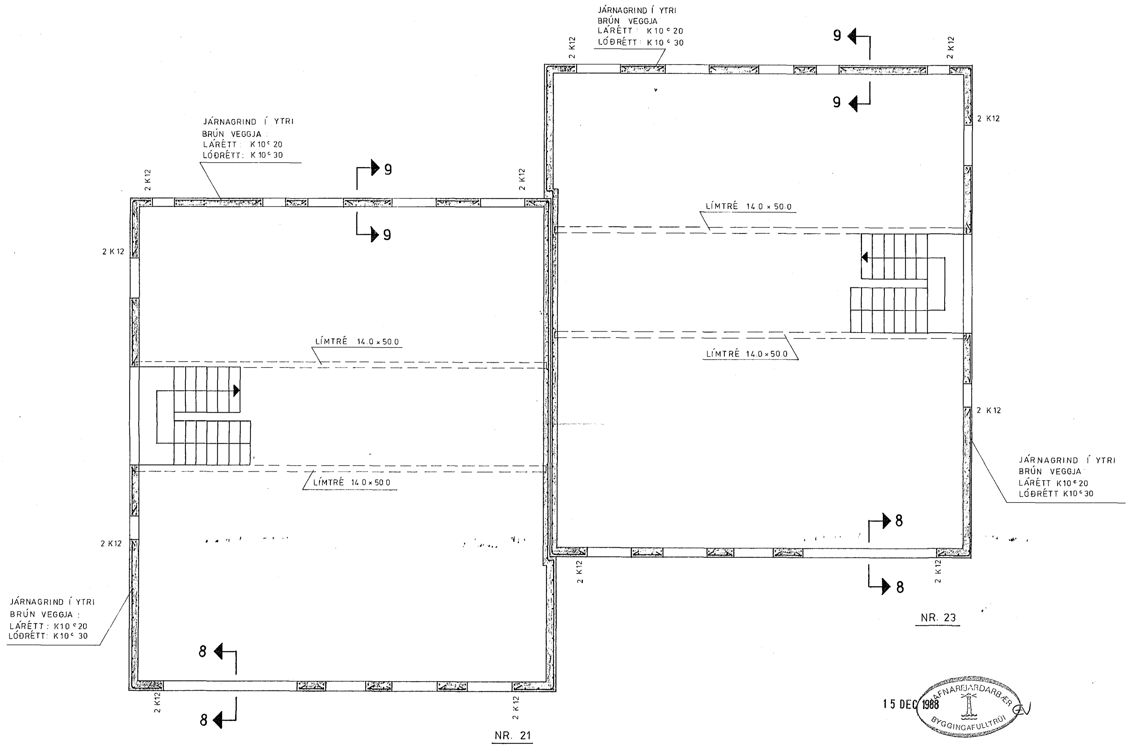
GRUNNMYND 1:50
