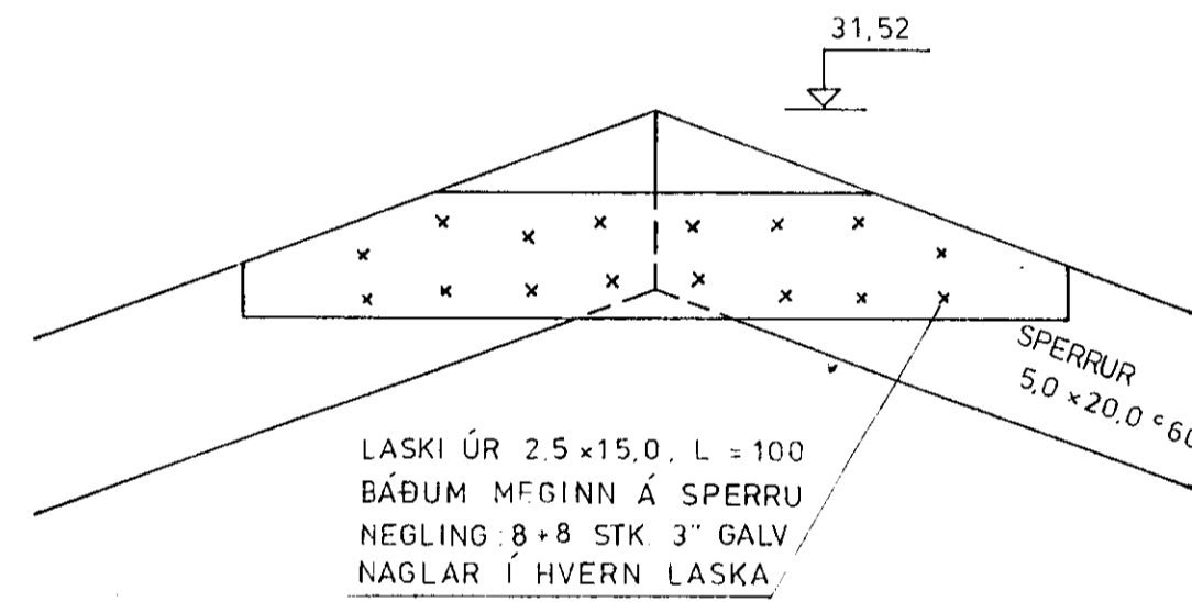
SÉRMYND C 1:10
