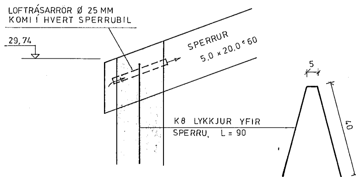
SÉRMYND B 1:10
