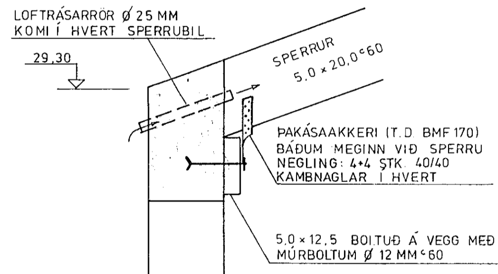
SÉRMYND A 1:10
