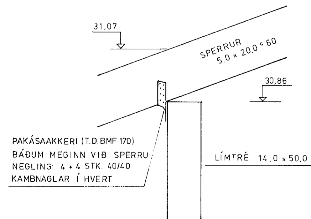
SÉRMYND D 1:10
