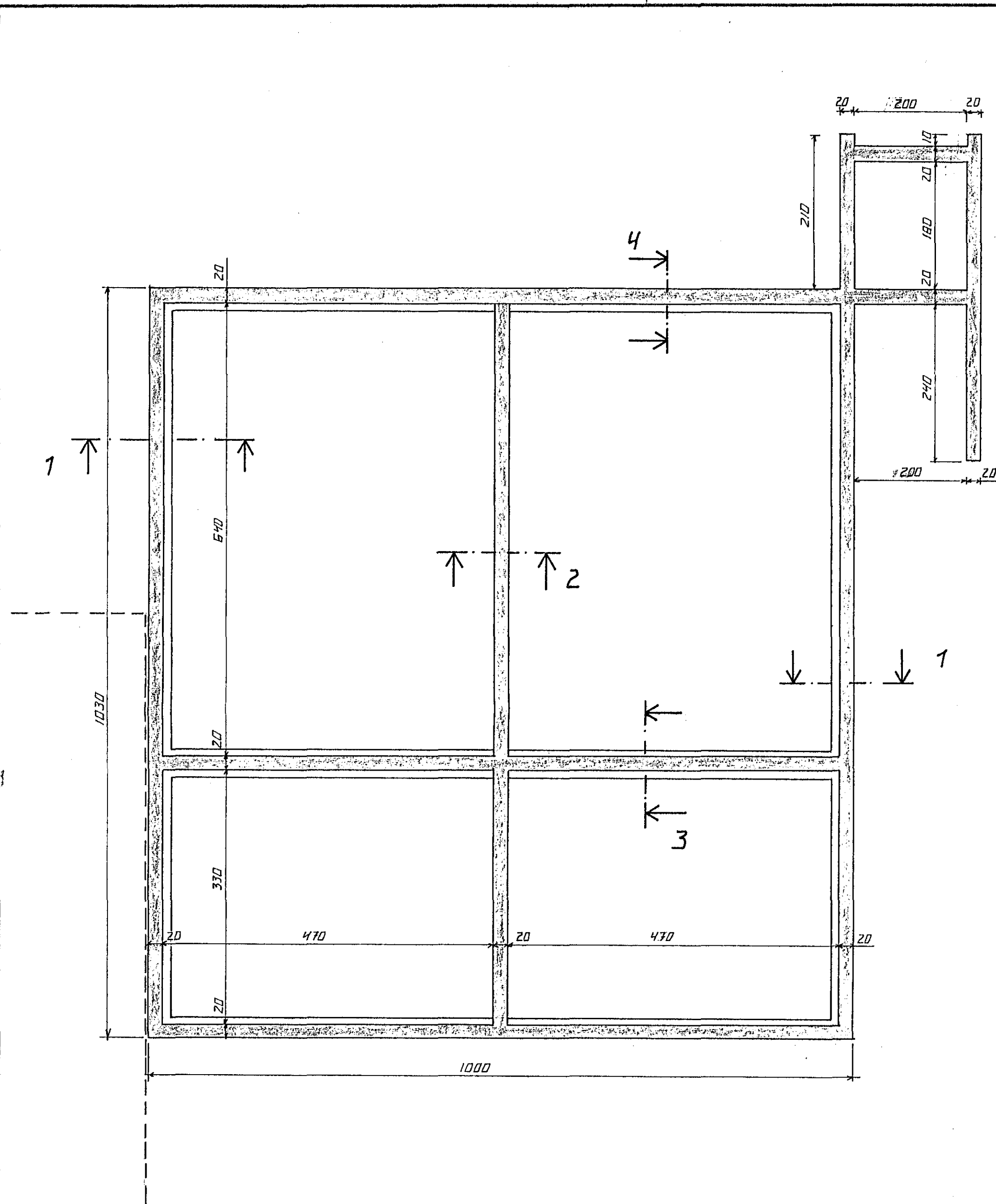
GRUNNMYND 1:50
