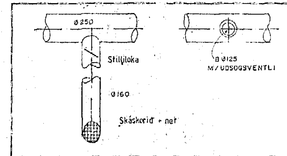
ÚTSOGSVENTLAR KENNISNIÐ 1:20
