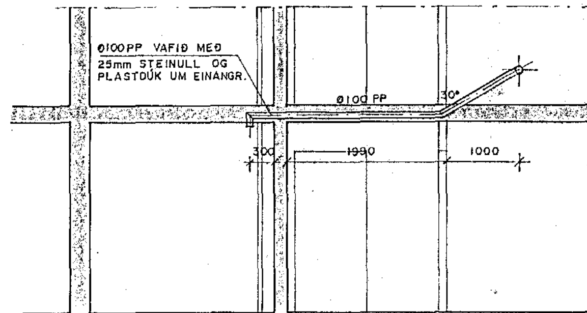
LOFTRÆSING F. ÞURRKARA 1:50
