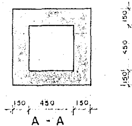
LOFTRÆSIOP Í LOFTPLÖTU 1:20
