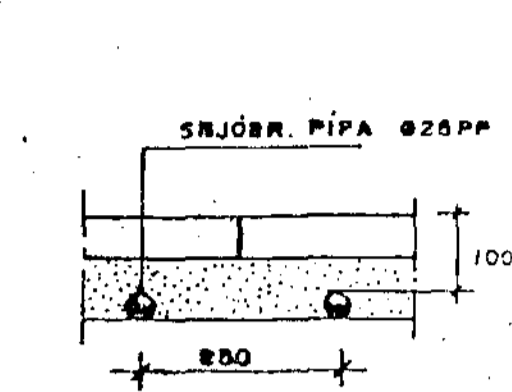
SNJÓBRÆÐSLA Í STÉTT 1:10
