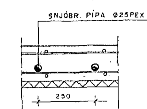
SNJÓBR. Í STEYPTRI GANGSTÉTT 1:10
