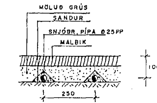
SNJÓBRÆÐSLA Í MALBIK 1:10
