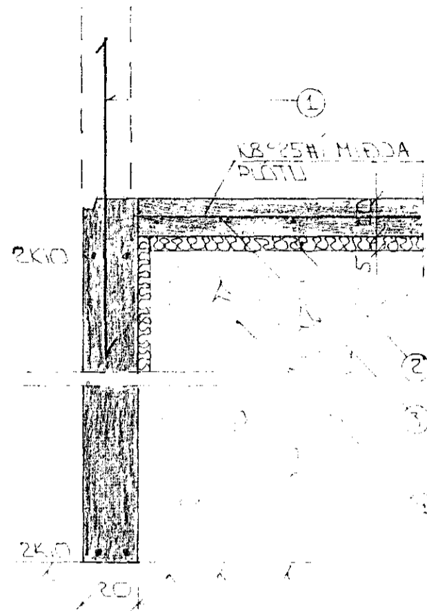
SNIB 1 Í ÚTVEGGI 1:20
