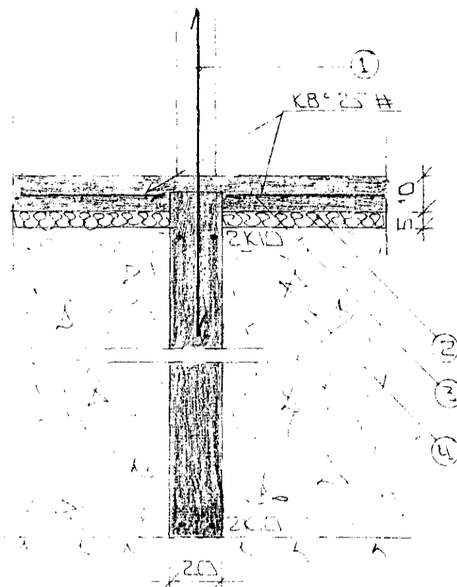
SNIB 3 Í MILLIV. 1:20
