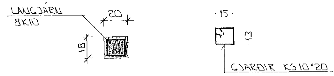
SÚLA S1 + 1:20
