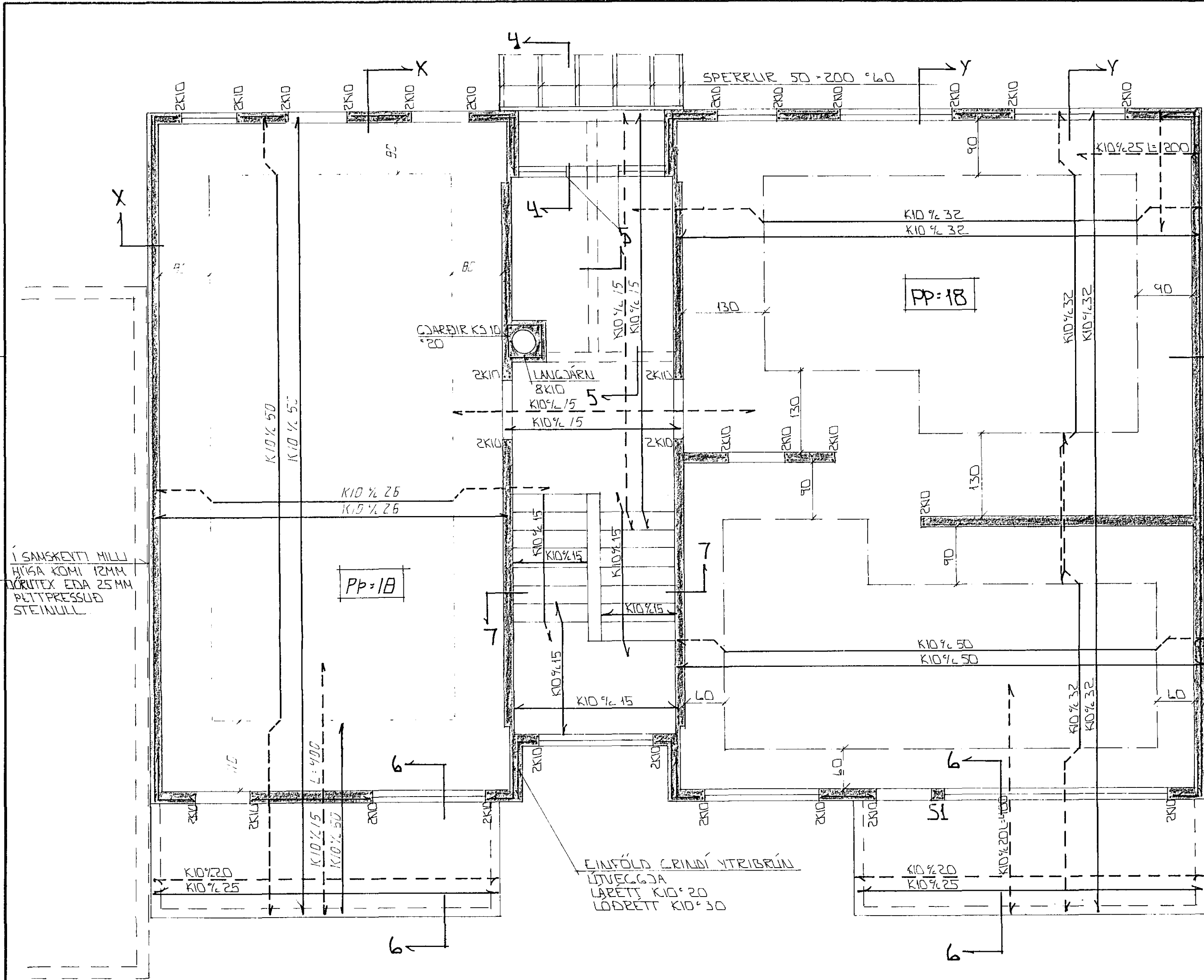
GRINDMYND + 1:50
