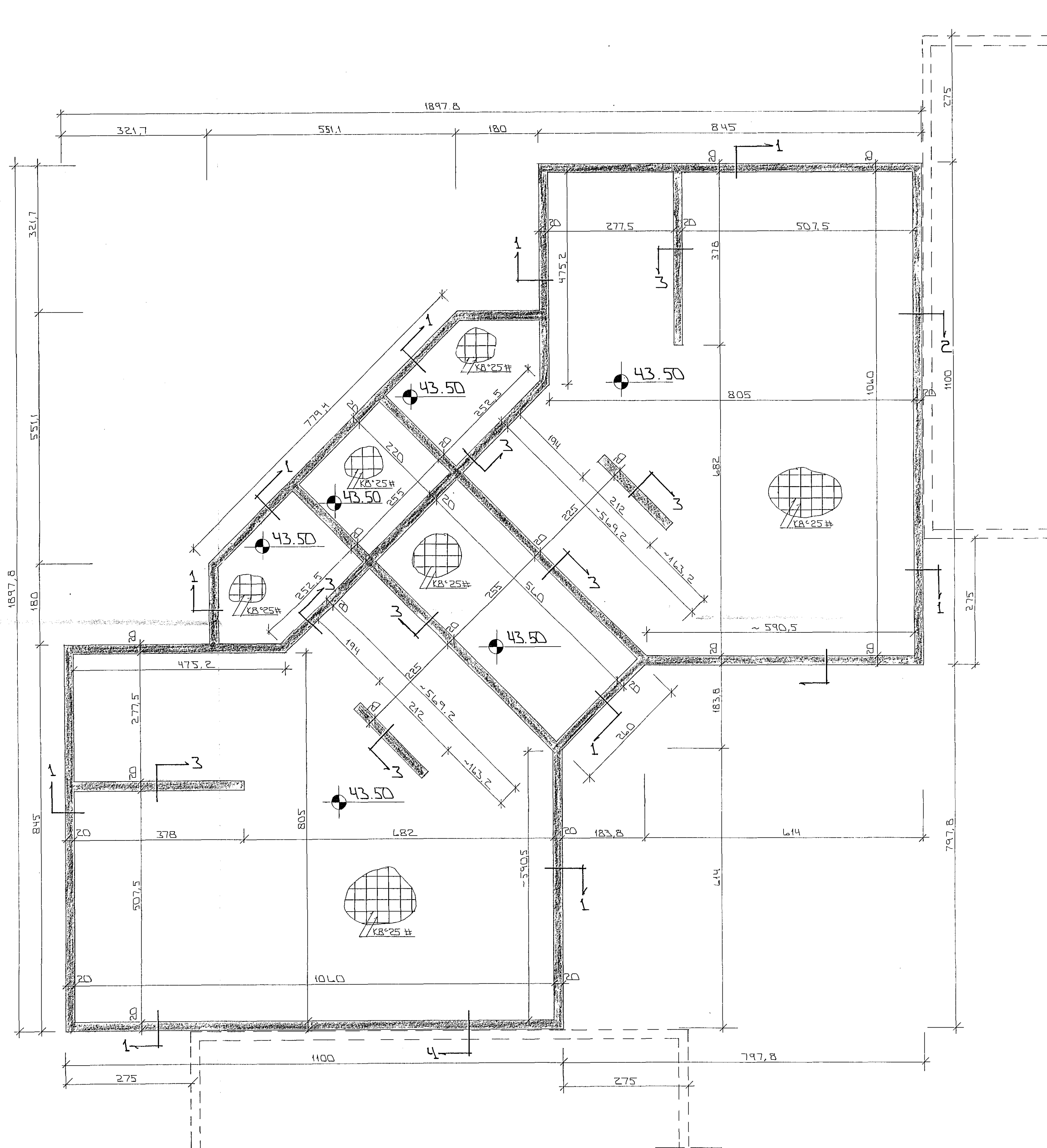
CRUNNMÝND 1:50
