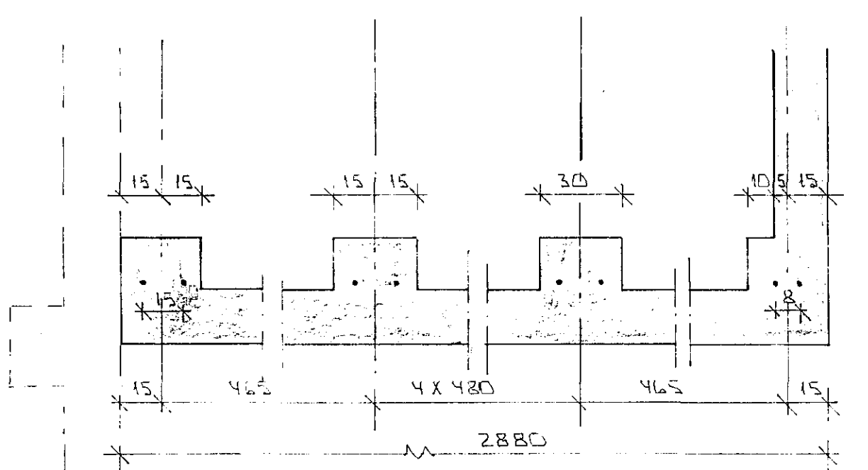
STADSETNING BOLTA FYRIR RAMMA 1:20 SÁ NÁRAR TEKN. FRAML.
