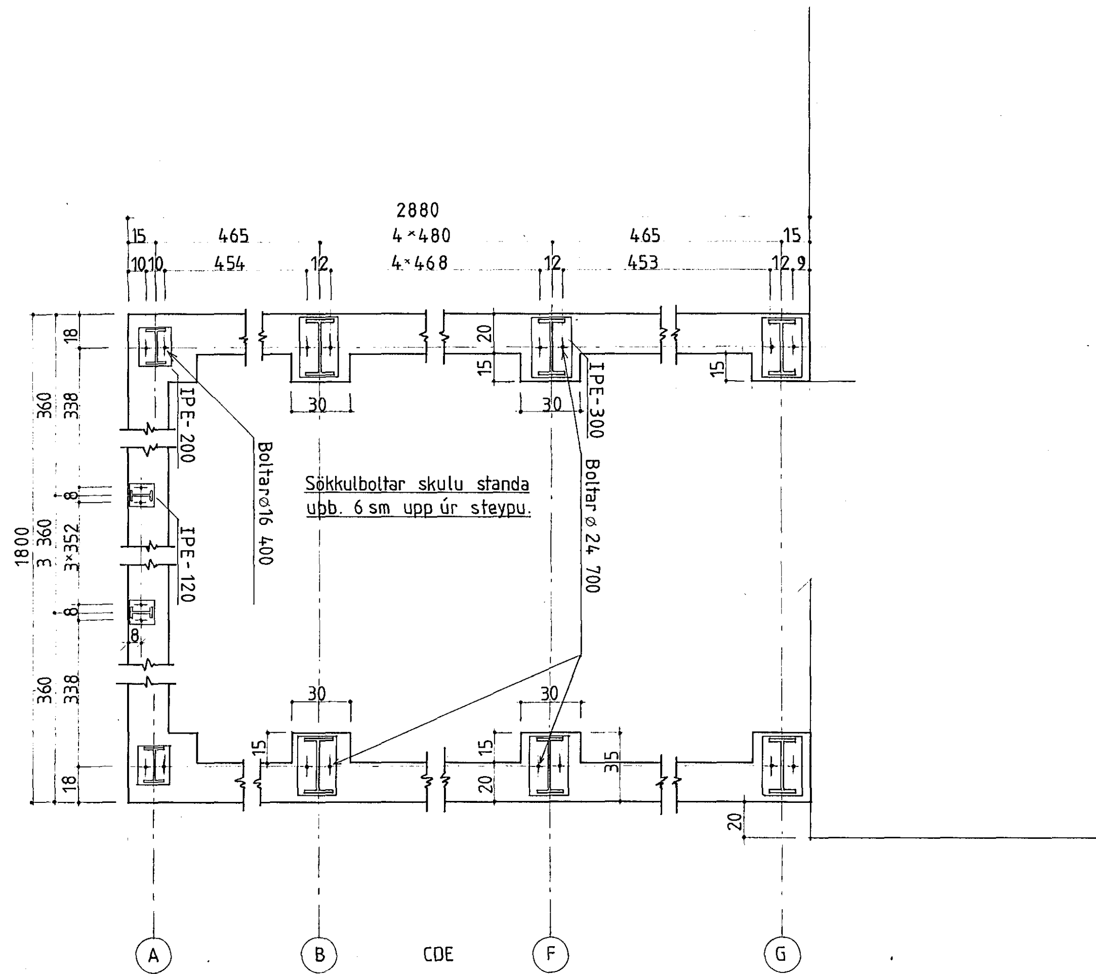
SÖKKUL-, BOLTATEIKNING MKV. 1:20
