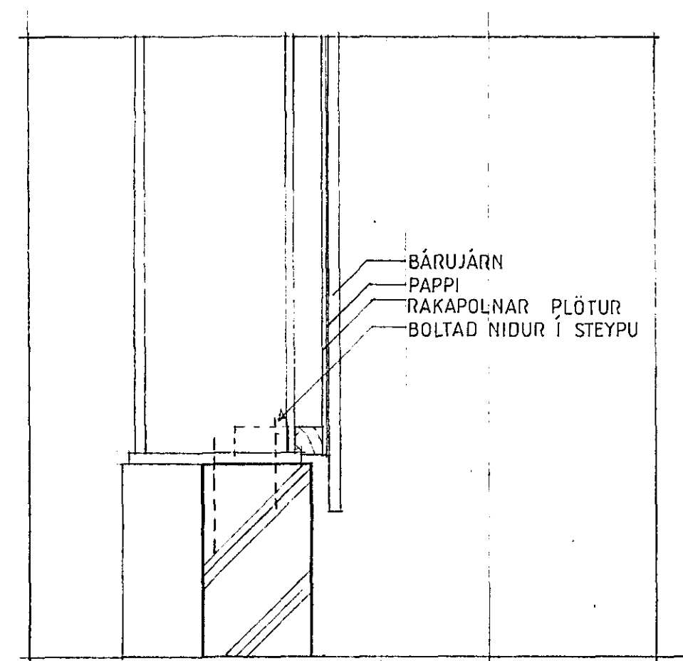
HLUTATEKNING A MKV. 1:10
